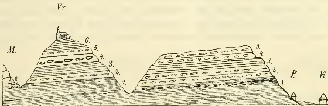
Fig. 40. Profil von Vinar nach Vraclav (unweit Hohenmanth). Vi. Vinar. P. Pazderna. Vr. Vraclav. M. St. Niclas. 1. Semitzer Mergel. 2. Dřinover Knollen. 3. Wehlowitzer Fischpläner und Malnitzer Schichten. 4. Byšicer Uebergangs-Schichten mit Halec Sternbergii . 5. Tiefere Lagen der Trigoniaschichten. 6. Höhere Lagen der Trigoniaschichten mit Callianassa und Hemiaster plebeius .
