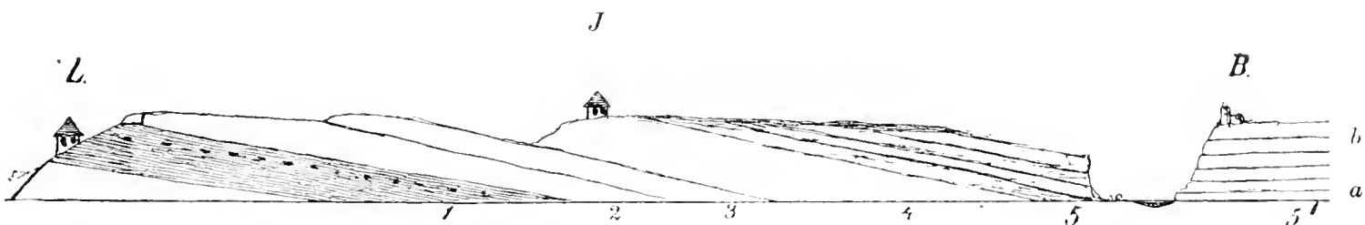
Fig. 20. Profil von Lisa (L) nach Benatek (B).
