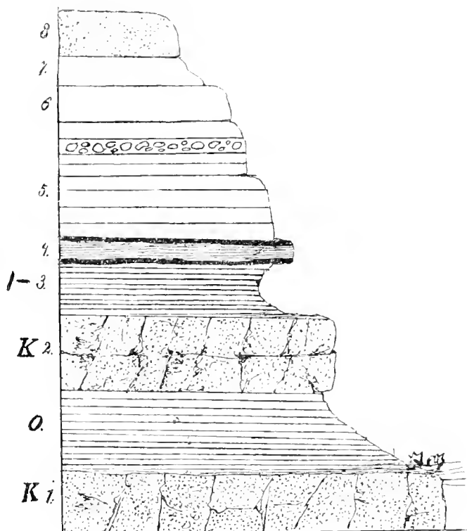
Fig. 19. Profil der Thallehne gegenüber Kadlin. K1 . Erster Kokořiner Quader in der Thalsole verdeckt. O . Zwischenpläner. K2 . Zweiter Kokořiner Quader. 1.—8. Lagen der Trigoniaschichten, mit denen von Choroušek (p. 30) übereinstimmend.
