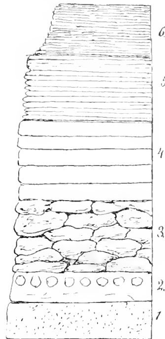
Fig. 44. Profil im Steinbruche „Na Libánkách“ bei Leitomischel (aufgenommen im Jahre 1867.) 1. Sandige Lage. 2. Lage mit Exogyra . 3. „Havle“-Kalkstein ohne regelmässige Lagerung mit Callianassa . 4. „Hlavní Pecina“, guter Baustein mit zahlreichen senkrechten Fucoidenstängeln . 5. „Pecina“-Baustein, zweite Kategorie. 6. Rumovka oder Sadrák ( Bryozoenschichten ).
