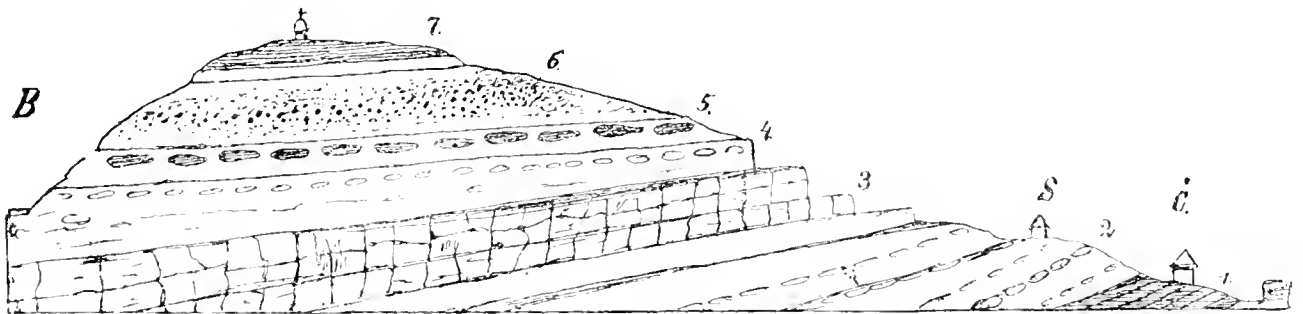
Fig. 14. Profil zwischen Byšic und Čečelic. B. Balm bei Byšic. Č. Čečelic. S. Schüttboden. 1. Semitzer Mergel mit zahlreichen Petrefacten beim nahen Orte Všetat. 2. Dřinover Knollen mit Lima elongata . 3. Wehlowitzer Pläner in einem Steinbruche gut entblösst. 4. Malnitzer Schichten. 5. Grosse Knollen mit Fischschuppen. Byšicer Uebergangsschichten. 6. Rostrothe Sande (Aequivalente der beiden Kokořiner Quader). 7. Die tiefsten Lagen der Trigoniaschichten (mit grossen Inoceramus Brongniarti ).
