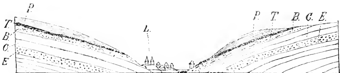
Fig. 43. Profil bei Leitomischel (L) in der Richtung von Osten nach Westen. E. Trigoniaschichten mit grossen Exogyra conica . C. Desgleichen mit zahlreichen Scheeren von Callianassa antiqua . B. Bryozoenschichten (Sadrák). T. Blaue Thone mit Terebratula subrotunda (Teplitzer Schichten). P. Priesener Schichten.
