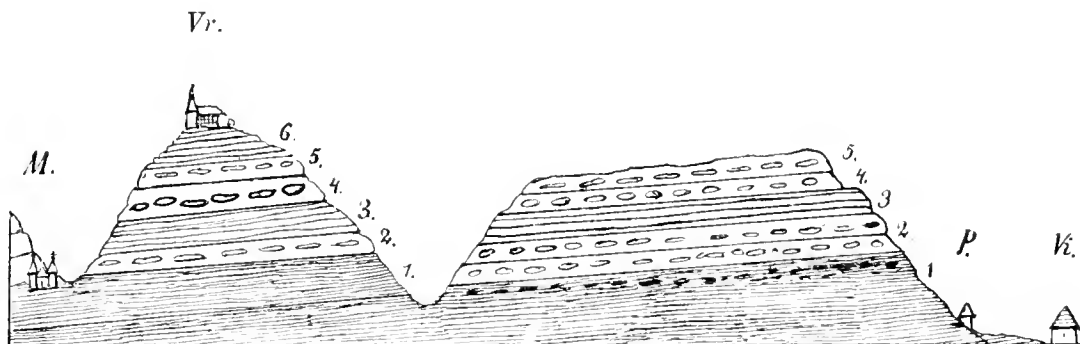
Fig. 40. Profil von Vinar nach Vraclav (unweit Hohenmauth). Vi. Vinar. P. Pazderna. Vr. Vraclav. M. St. Niclas. 1. Semitzer Mergel. 2. Dřinover Knollen. 3. Wehlowitzer Fischpläner und Malnitzer Schichten. 4. Byšicer Uebergangs-Schichten mit Halec Sternbergii . 5. Tiefere Lagen der Trigoniaschichten. 6. Höhere Lagen der Trigoniaschichten mit Callianassa und Hemiaster plebeius .
