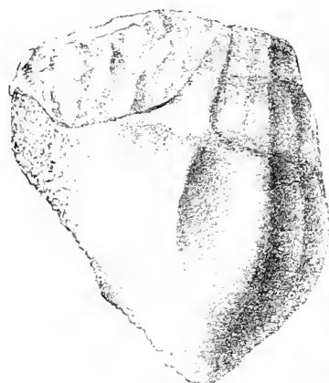
Fig. 60. Rostellaria Schlottheimi von Chotzen. Nat. Gr.
