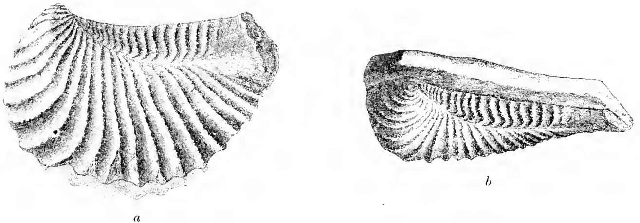
Fig. 66. Trigonía limbata d'Orb. Nach einem Gypsabgüsse in das Negativ aus der Gegend von Böhm.-Trübau. Nat. Grösse. a von der Seite, b von Oben.
