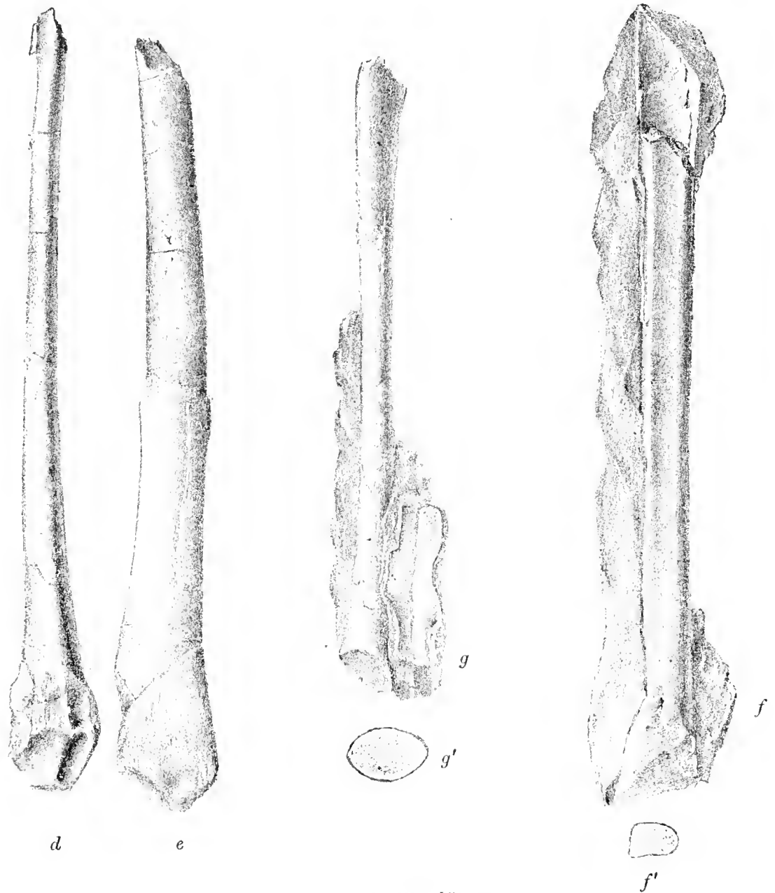
Fig. 45. Cretornis Hlaváči , Fr.
