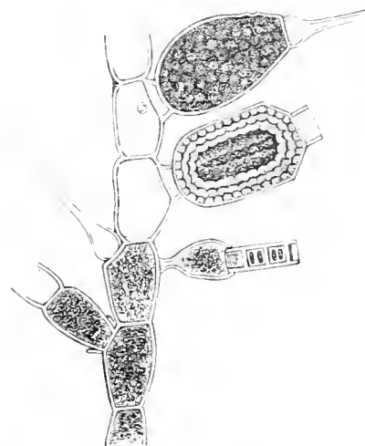
Fig. 17. Bulbochaete rectangularis Wittr. Stück eines Fadens mit einem noch nicht befruchtetem, und einem eine entleerte Oospore mit längs geripptem Epispor enthaltenden Oogonium, sowie mit einem Zwergmännchen unter d. letzteren Oogonium. Vergr. etwa 300mal.
