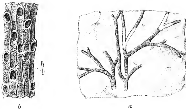
Fig. 106. Entalophora Geinitzii Reuss. a Aus den Bryozoenschichten von Vtelno, in nat. Grösse. b Vergrössert.
