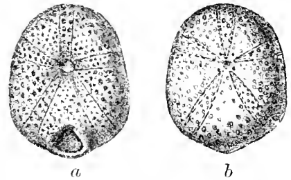
Fig. 124. Caratomus Laubei Nov. aus den Bryozoen-Schichten v. Vtelno. a Von unten, b von oben 2mal vergrößert.
