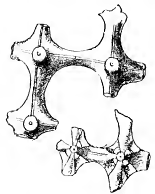
Fig. 28. Nadeln in dieser Höhlung gefunden.
