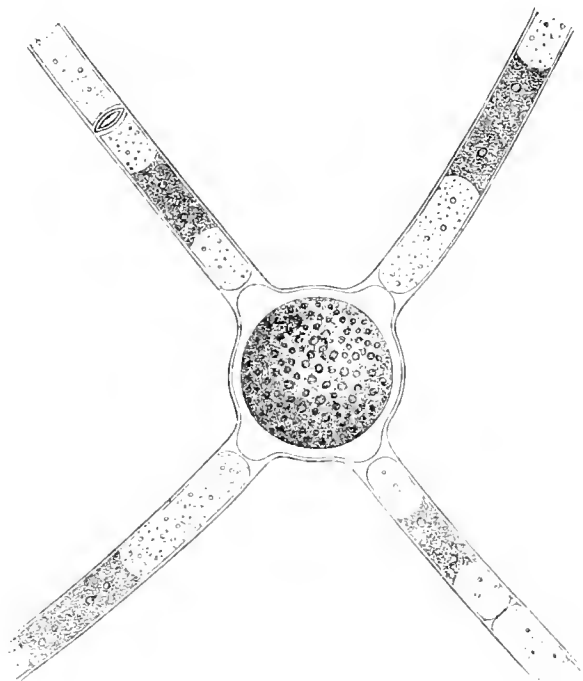
Fig. 94. Mougeotia corniculata nob. Stück eines copulirten Fadenpaares, mit einer fast reifen Zygote, etwa 500mal vergr.
