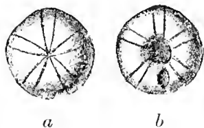
Fig. 117. Holotypus Turonensis Desor. aus den Bryozoenschichten von Živonín. Nat. Grösse. a Von oben, b von unten.
