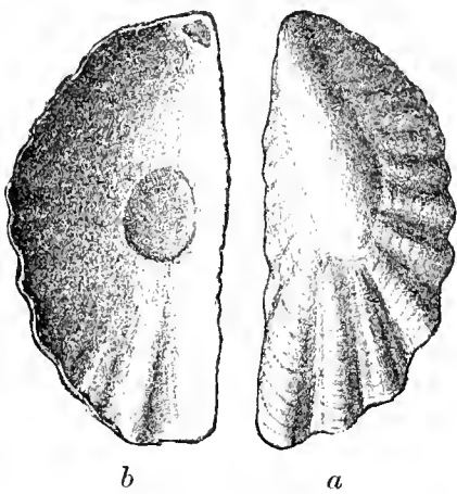
Fig. 96. Ostrea frons Park. aus den Bryozoen-schichten v. Živonín. 2mal vergrößert. a Oberschale von oben, b dieselbe von innen.
