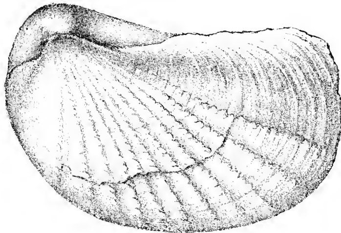
Fig. 76. Pholadomya nodulifera M. von Jungbunzlau. Nat. Grösse.
