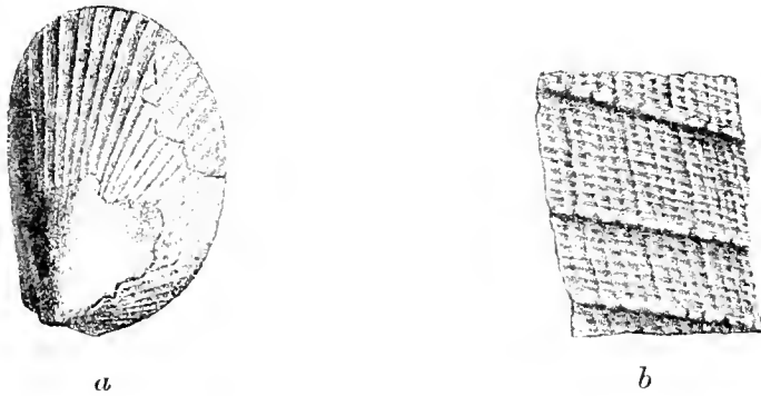
Fig. 85. Lima ovata Römer? von Böhm.-Trübau. a Nat. Grösse. b Schale vergrössert.
