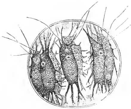
Fig. 50. Stephanosphaera pluvialis Cohn. Eine achtzellige Familie in Aequatorialansicht. Die Primordialzellen sind mit zahlreichen Hauffäden versehen. Vergr. etwa 600fach. (Nach Hieronymus.)
