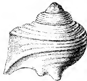
Fig. 59. Rostellaria ovata , Münst. Von Třeboutic.
