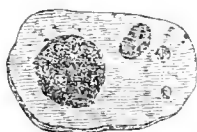
Fig. 5. Hildenbrandtia rivularis (Liebm.) J. Ag. Von Eisenbrod. Vier kleine an einem Kieselstein-Bruchstück angewachsene Exemplare. (Nat. Grösse.)
