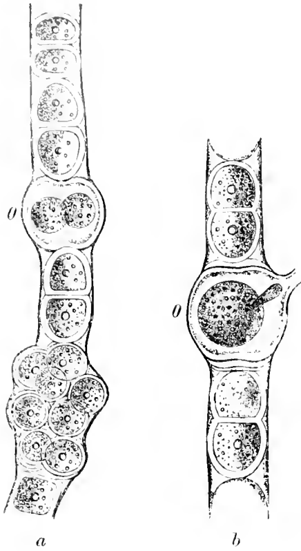
Fig. 122. Cylindrocapsa geminella Wolle var. minor nob. a) Theil eines Oogonien tragenden Fadens, o ein Oogonium nach erfolgter Zweitheilung der Oosphäre; b) Fadenbruchstück mit einem geöffneten Oogonium o . Vergr. etwa 500m.
