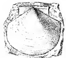
Fig. 88. Pecten Nilsoni Gein. aus den Trigoniaschichten von Böhm.-Trübau. Nat. Grösse.
