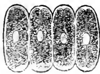
Fig. 61. Scenedesmus bijugatus (Turp.) Ktz. ( S. obtusus Meyen). Eine vierzellige Familie mit 3 sich theilenden Zellen (600fach vergr.).
