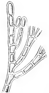
Fig. 42. Chlorotylum cataractarum b) incrustans. Endtheil eines verästelten Fadens, etwa 250fach vergr.
