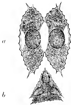
Fig. 120. Staurastrum denticulatum (Näg.) Arch. a) Eine Zelle in der Längsansicht, 600-fach vergr.; b) in der Queransicht, 300fach vergr.
