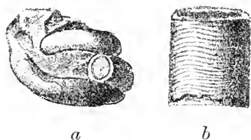
Fig. 114. Serpula ampulacea Sow. von Choroušek. a Nat. Grösse, b Fragment d. Schale vergrössert, die Mittelschicht zeigend.
