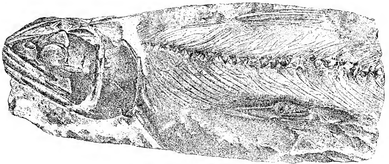
Fig. 47. Halec Sternbergii , Ag. von Jung-Koldin, etwa \frac{1}{3} nat. Grösse.
