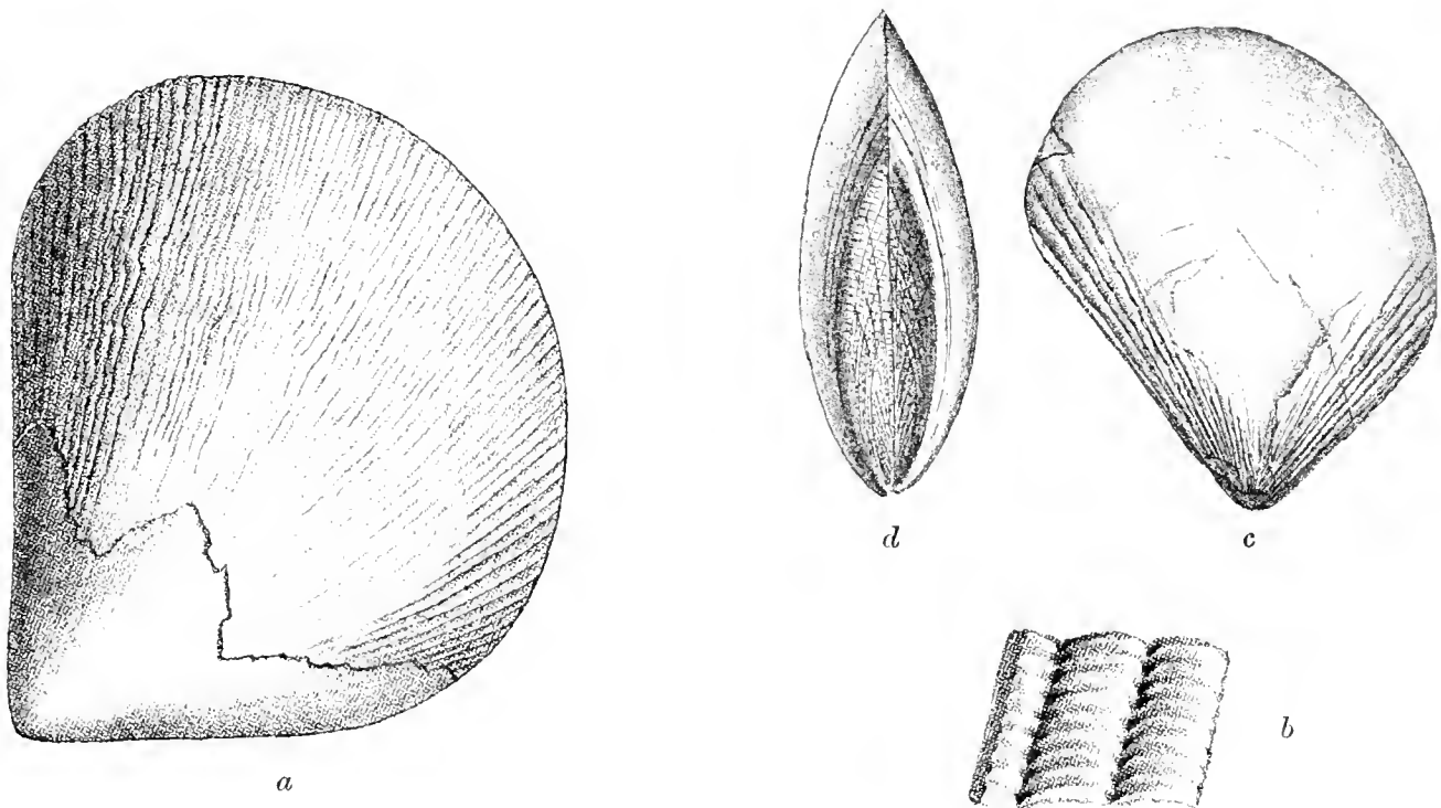
Fig. 86. Lima dichotoma Reuss. a Grosses Exemplar in nat. Grösse von Chotzen. b Fragment der Schale desselben Exemplars vergrössert. c Kleines Exemplar mit spärlicher Streifung in nat. Grösse von Chotzen. d Dasselbe von vorne.
