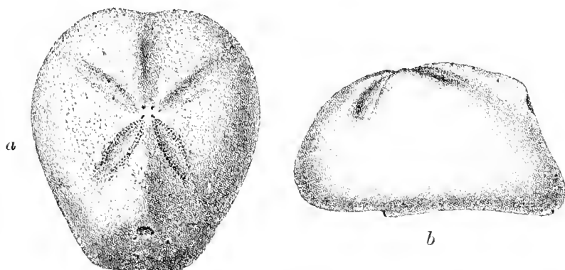
Fig. 119. Micraster Michelini Ag. Steinkern aus den Trigoniaschichten von Chotzen. Nat. Gr. a Von oben, b von der Seite.
