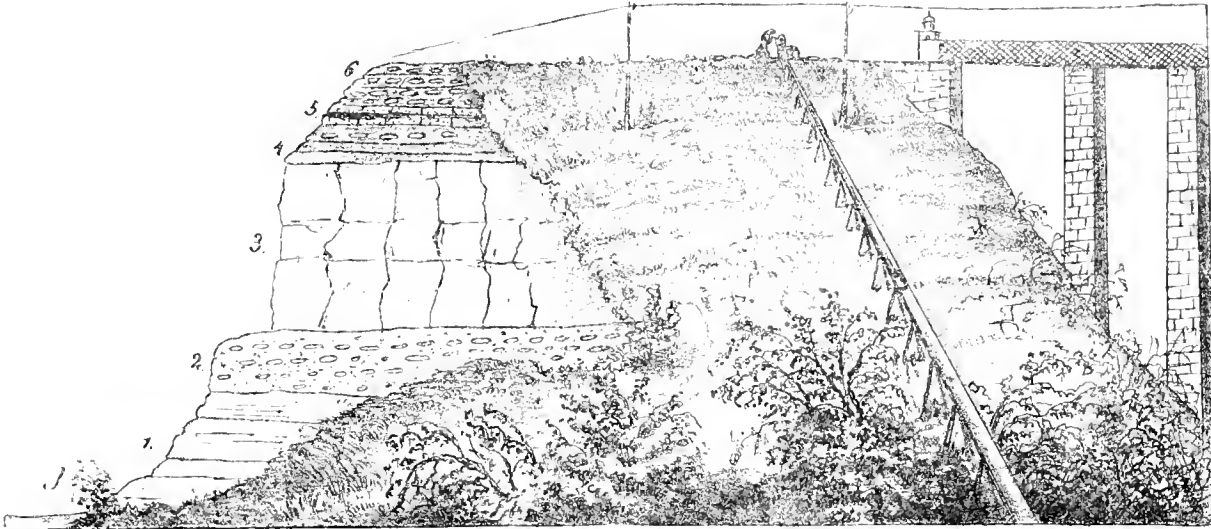
Fig. 22. Profil der Lehne des Iserthales beim Viaducte in Záměstí nad Ohří (Station Krnsko-Stranov). (J.) Iserfluss. 1. Tiefste Lagen der Trigoniaschichten. 2. Bank mit grossen Exogyra conica . 3. Podvinecer Baustein. 4. Sandige Knollenpläner mit zahlreichen Serpula socialis . 5. Zwei schwache Quaderbänke durch Plänerlagen getrennt. 6. Die höchsten Lagen der Trigoniaschichten (vielleicht schon Bryozoenschichten).
