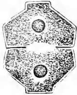
Fig. 115. Cosmarium salinum nob. Eine veget. Zelle im breiten Seitenprofil, etwa 500mal vergr.
