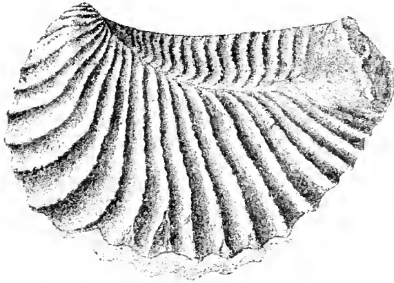
Fig. 7. Trigonina limbata . D'Orb.
