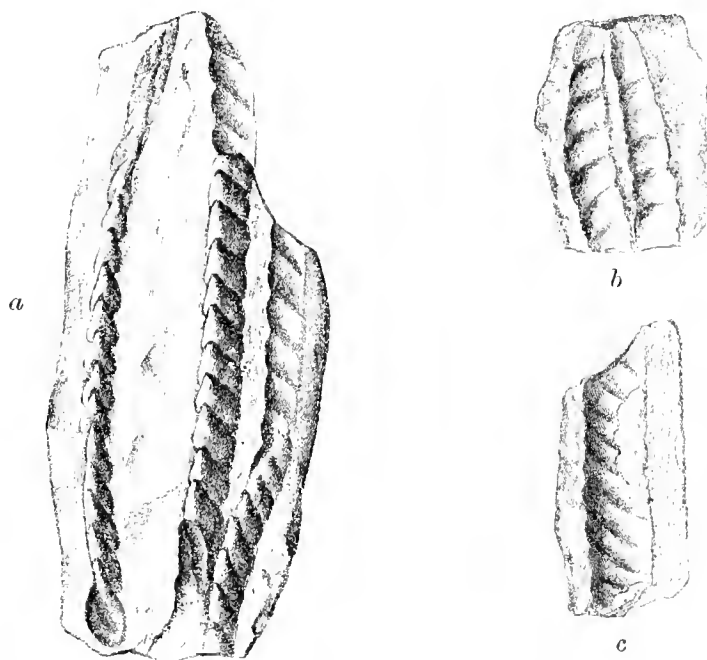
Fig. 132. Fucoïdes? strangulatus Fr. a Aus den Trigoniaschichten von Leitomischel, b von Choroušek, c von Schellesn. Nat. Grösse.
