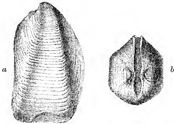
Fig. 61. Opis Chocenensis Fr. von Chotzen. Nat. Gr. a Von der Seite, b von oben.
