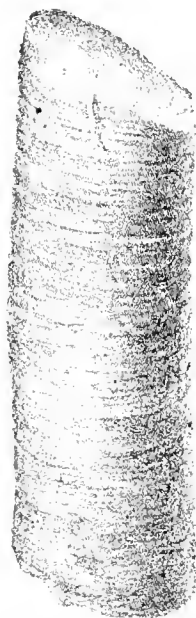
Fig. 130. Fucoïdes columnaris Fr. Fragment in nat. Gr. von Chotzen.
