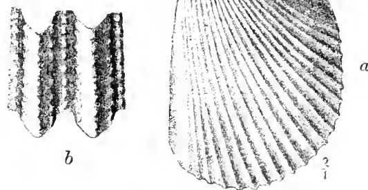
Fig. 84. Lima iserica Fr. n. sp. Aus den Trigoniaschichten von Brandeis an der Adler. a 2mal vergrössert, b Fragment der Schale stark vergrössert.
