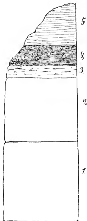
Fig. 34. Schema der Schichtenfolge bei Abtsdorf.
