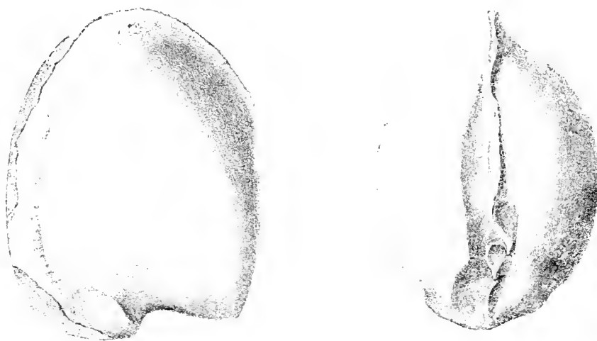
Fig. 65. Cyprina quadrata , d'Orb. Steinkern von Chotzen. \frac{1}{2} nat. Grösse.
