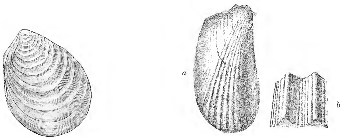
Fig. 80. Inoceramus Brongniarti . Steinkern aus den tieferen Lagen der Trigonia-schichten bei Jungbunzlau. \frac{1}{10} nat. Grösse.
