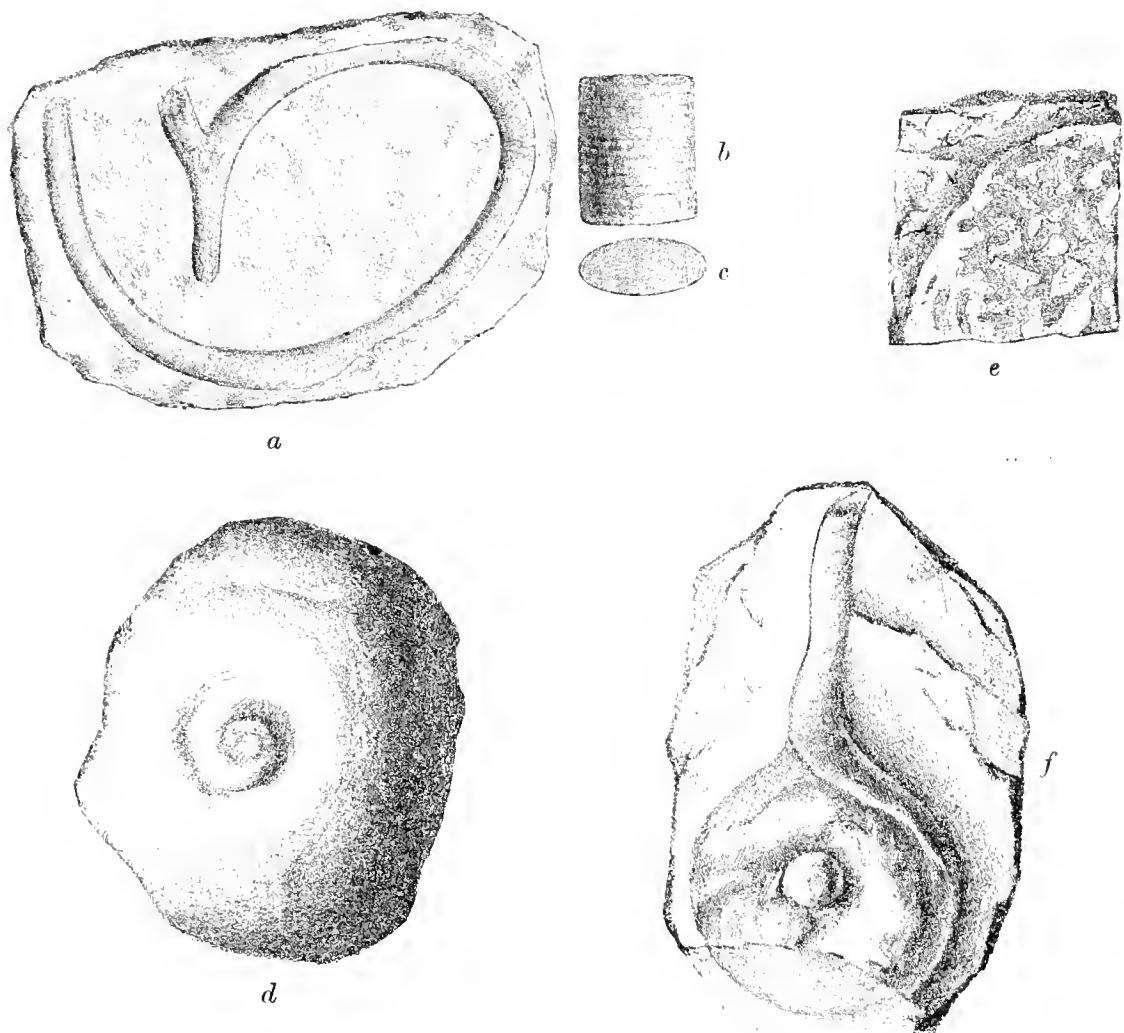
Fig. 129. Fucooides funiformis Fr. a Ein sich verzweigender strickförmiger Ast, \frac{1}{4} nat. Grösse. b Fragment desselben mit Querrunzeln, nat. Grösse. c Querschnitt, nat. Grösse. d Wurzelhöcker mit Nabel von oben, nat. Grösse. e Schwammige Basis des Höckers. f Ein genabelter Höcker, von dem ein strickförmiger Ast entspringt, \frac{1}{2} nat. Gr. (Alles aus den tieferen Trigoniaschichten beim Friedhofe in Chotzen.)
