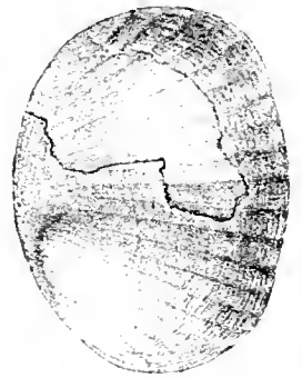
Fig. 99. Anomia? sp. aus dem Sandstein v. Auscha. 2mal vergrössert.
