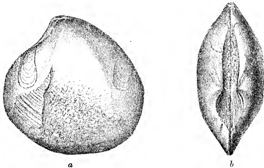
Fig. 78. Cytherea polymorpha Zittel. Steinkern aus den Trigoniaschichten von Písnik. Nat.-Gr. a Seitenansicht, b von oben.
