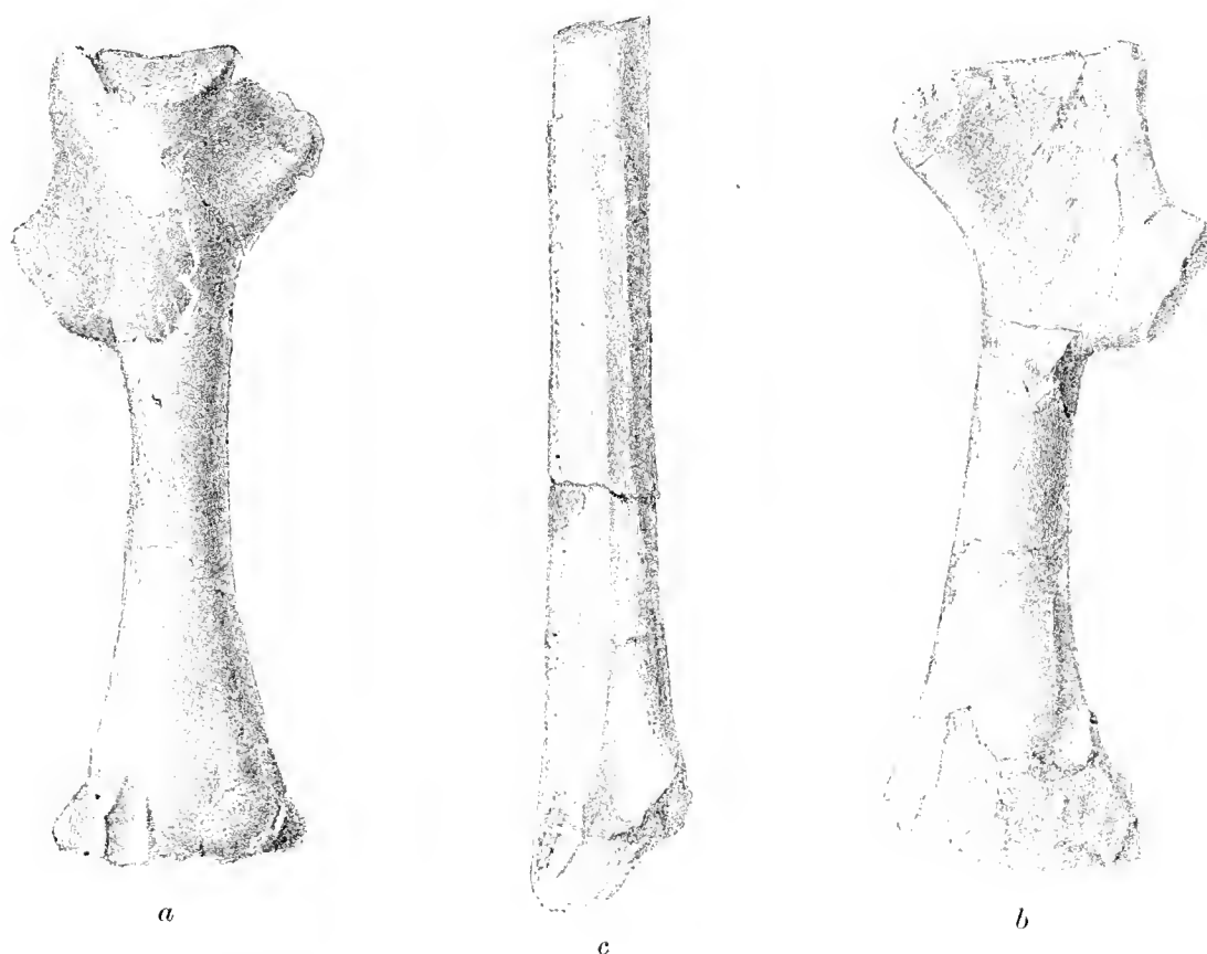
Fig. 45. Cretornis Hlaváči , Fr.
