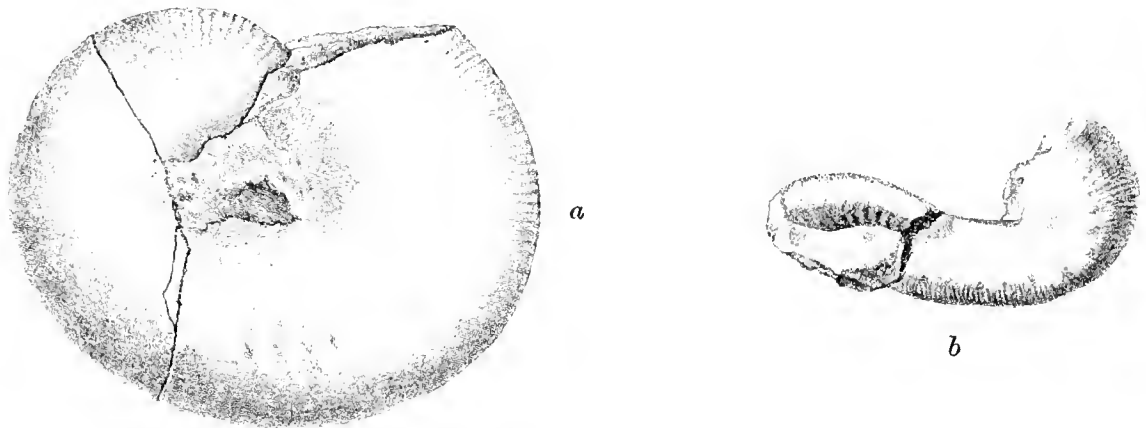
Fig. 53. Scaphites Geinitzii , d'Orb.
