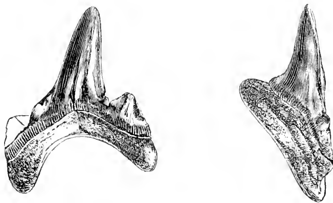
Fig. 46. Otodus semiplicatus , Münst. Nat. Grösse.
