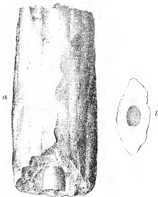
Fig. 131. Fucoïdes cauliformis Fr. a Fragment mit ausgefüllter Höhlung von Choroušek, nat. Grösse. b Querschnitt.
