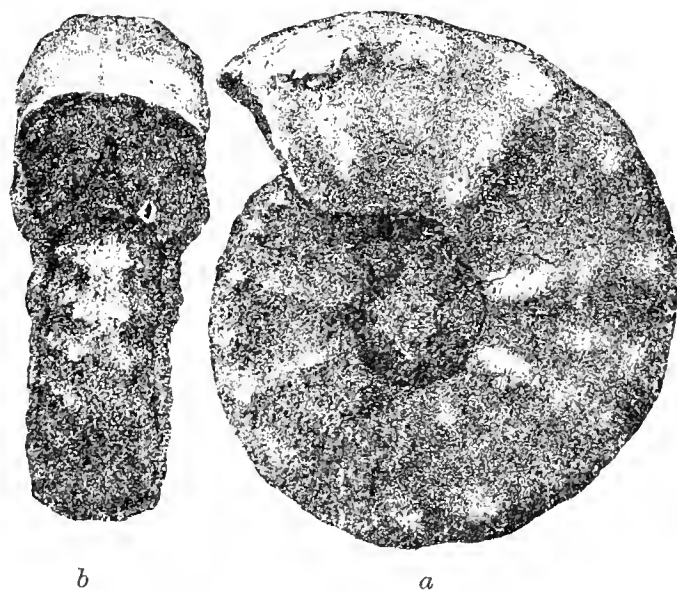
Fig. 52. Ammonites conciliatus , Stol. Aus den Iersschichten von Böhm.-Trüban. \frac{1}{3} nat. Grösse. a von der Seite. b von Vorne.
