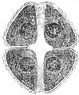
Fig. 116. Cosmarium botrytis (Bory) Menegh. var. emarginatum nob. Eine veget. Zelle in der breiten Seitenansicht, etwa 400mal vergr.
