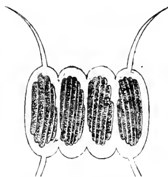
Fig. 62. Scenedesmus quadricauda (Turp.) Bréb. ( S. caudatus Corda). Eine vierzellige Familie, deren Zellen Brutfamilien erzeugen (600fach vergr.).
