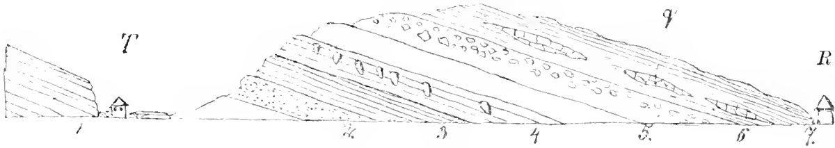
Fig. 32. Profil zwischen Triebitz (T) und Rybník (R).
