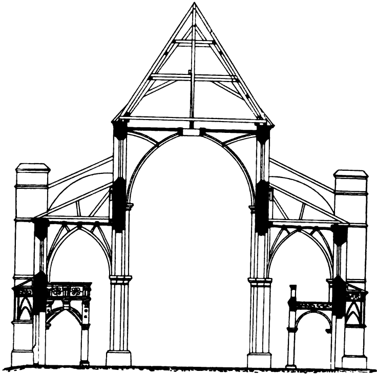
5. Querschnitt.
