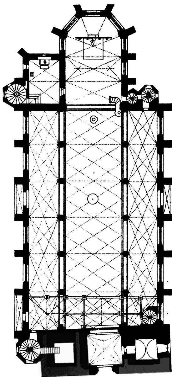
2. Grundriß.
