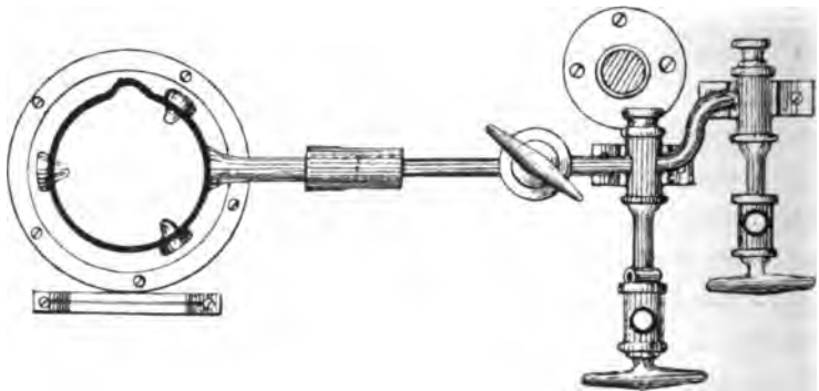
Fig. 2. Oberansicht des Apparates.
