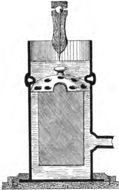
Fig. 1. Vertikaler Schnitt des Gefäßes.
