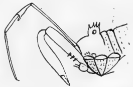
Fig. 45. Rhamsinitus filipes Rwr. — Cephalothorax des ♂ von links mit linker Chelicere und rechter Palpe.
