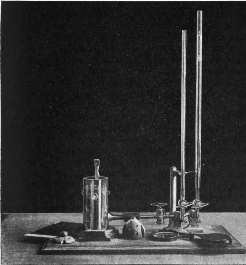
Fig. 3. Gesamtansicht des Apparates.
