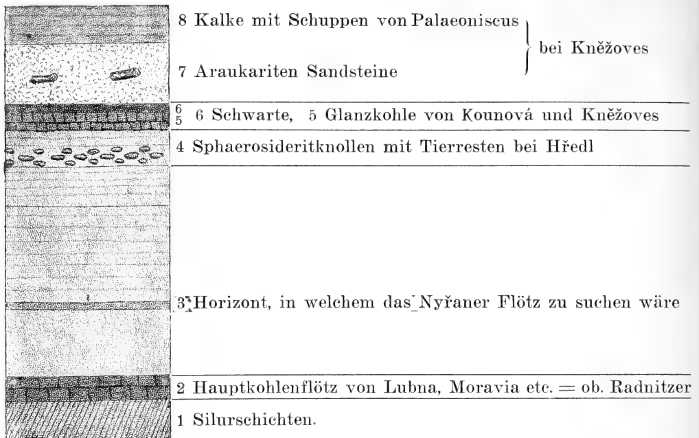
Fig. 33. Schematische Skizze der Schichtenfolge im Rakonitzer Becken.
