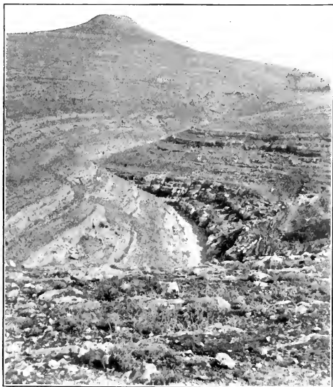
FIG. 39. GEBEL FUREIDIS.
