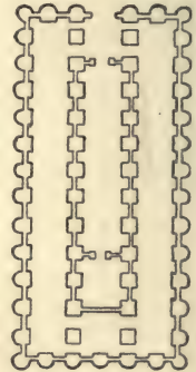
Fig. 7. PSEUDOPERIPTERAL.
