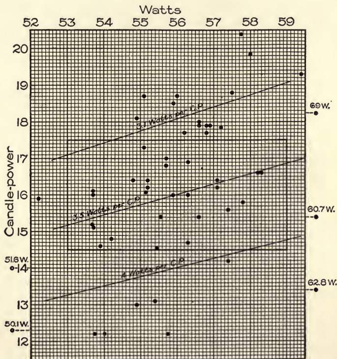
Fig. 37.—Shotgun Diagram.
