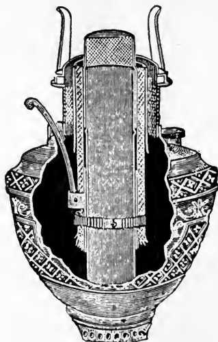
Fig. 17.—“Rochester” Kerosene Burner.
