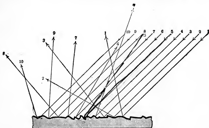
Fig. 11.—Diffuse Reflection.
