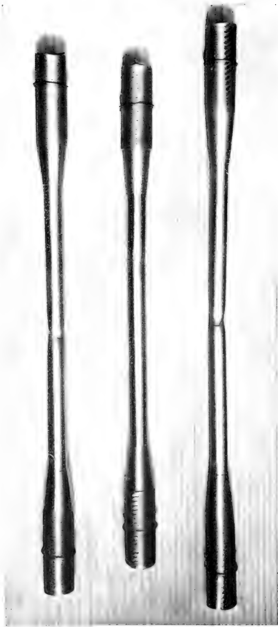
Prove di rottura a trazione su materiali ricotti a 800° (provette inizialmente identiche per forma e dimensioni). In alto: acciaio al 5% di nickel. — In mezzo: acciaio al 12% di nickel. — In basso: acciaio al 26% di nickel.
