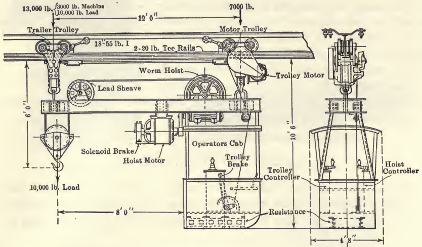
FIG. 307.—Telfer.
