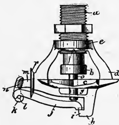
STAR SPRINKLER.
