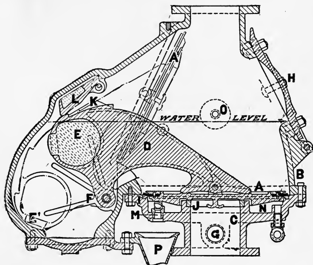
ROCKWOOD DRY VALVE A.
