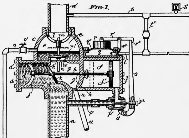
CLAPP DRY VALVE A.
