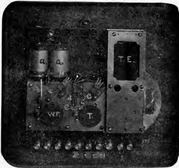
A. D. T. ALARM VALVE TRANSMITTER.
