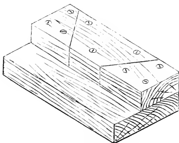
Fig. 8.—Mitre Block.
