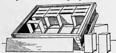
FIG. 129.— T-super.
