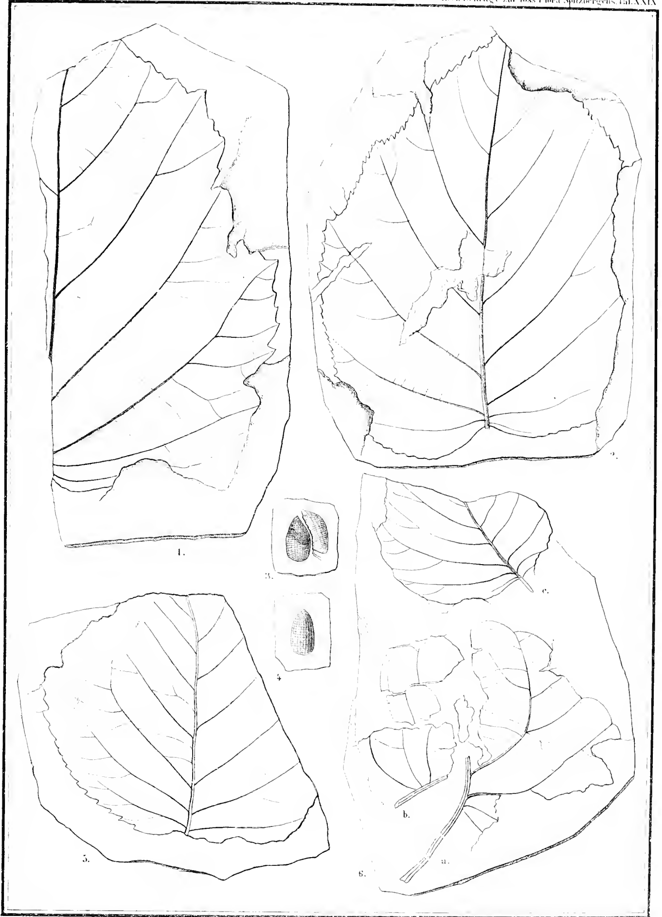
Fig. 1. Corylus Scottii. 2. Corylus M'Quarri microdonta. 3, 4. Nyssa reticulata. 5. Viburnum Nordenskiöldi. 6. Cornus ramosa.
