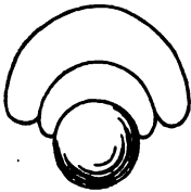
Fig. 7. Querschnitt d. Jugendwindungen von Neopt. telingaef. n. sp. 10/1.
