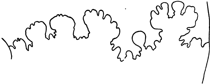
Fig. 48 Hopl. gibbosulus bipartitus (Taf. IV Fig. 10). a) Linke Suture und b) erster Laterallobus rechts bei 50 mm Windungsradius. 2/l.
