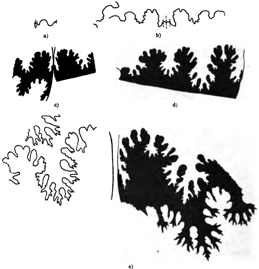
Fig. 17. Entwicklung der Lobelinie von Neopt. telingaef. var. discrepans n. var. von Balangl. Windungsradius: a) 0,5 mm, 15/1. b) etwa 5 mm, 6/1. c) etwa 15 mm, 4/1. d) 27 mm, 2/1. e) 42 mm, 2/1.
