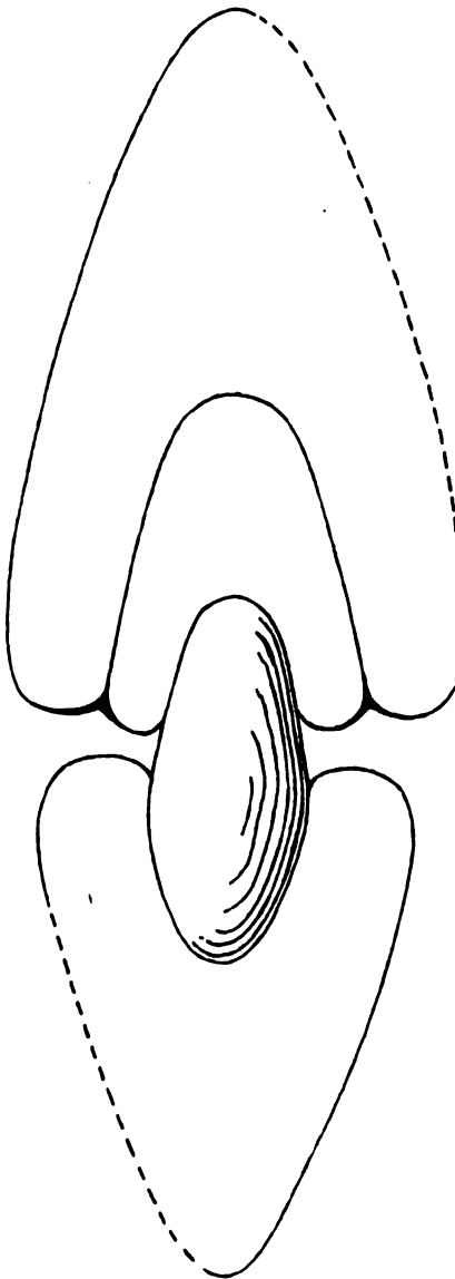
Fig. 8. Querschnitt eines erwachsenen Neopt. telsingaef. n. sp. (von dem auf Taf. III Fig. 2—4) abgebildeten Exemplar). Nat. Gr.
