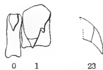
Radula von Pseudoglessula leroyi (Bgt.) 0 Mittelzahn, 1 erster Seitenzahn, 23 Randzahn.
