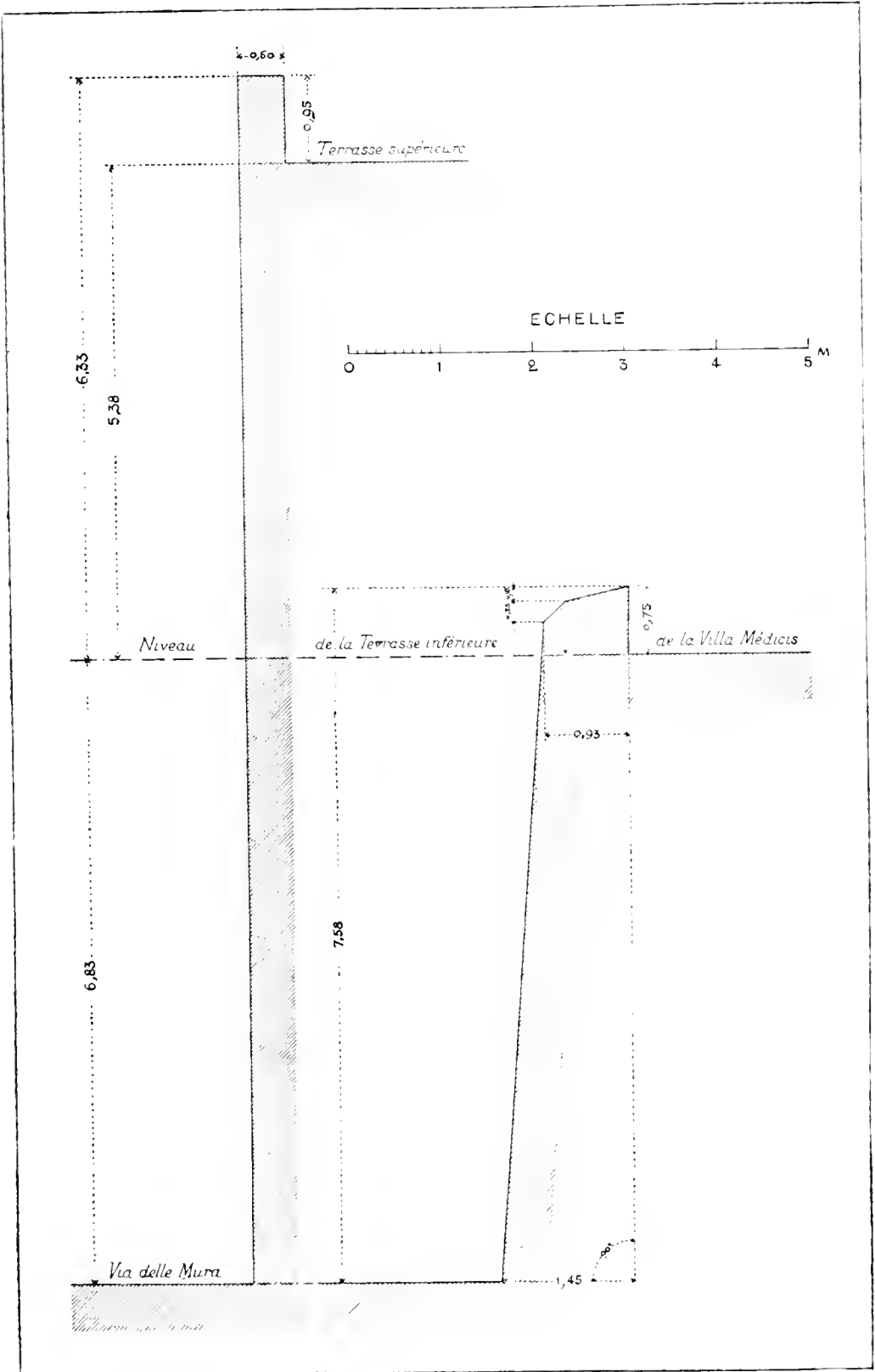
Fig. 17 et 18. -- Coupes de l'Encinte d'Aurélien, le long de la Villa Médicis.
