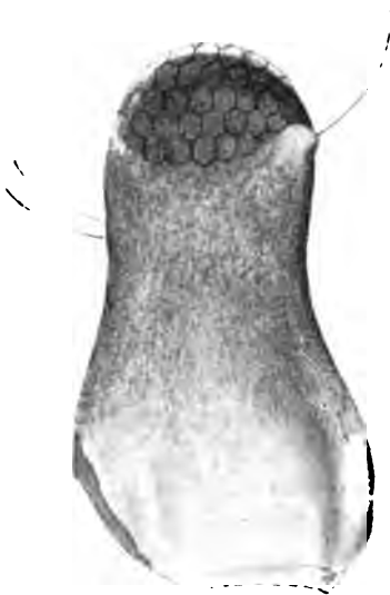
Physachaeus ctenurus. Auge von der Seite gesehen.
