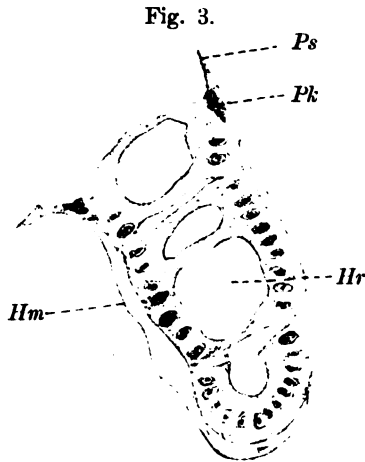
Lohmannia catenata , medianer Längsschnitt; Hämatoxylin. Vergr.: Leitz, Obj. 5, Oc. 1. Ps = Pseudopodium; Pk = Pseudopodienkern; Hr = Innerer Hohlraum eines Segmentes; Hm = Hüllmembran.
