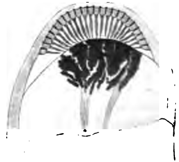
Schnitt durch das Auge von Ethusina abyssicola .
