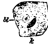
Secernierende Zelle des adipoiden Drüsengewebes der Hinterleibsspitze von Paussus cucullatus . (Zeiss Apochr. 2.0, 1.30 \times Compensoc. 6; 750:1.)
