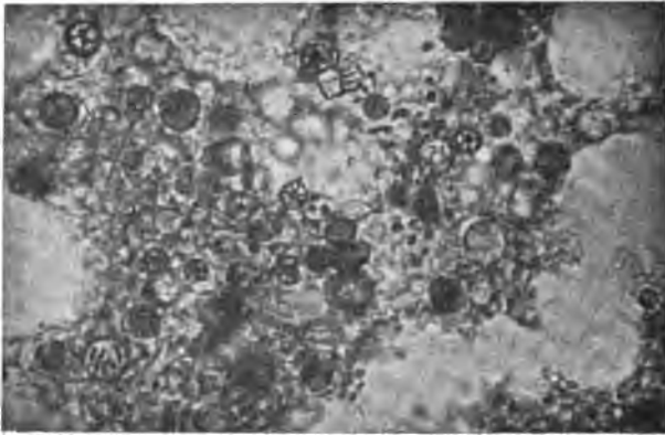
Schnitt durch das abdominale Fettgewebe einer Larve von Orthogonius Horni (800 : 1).
