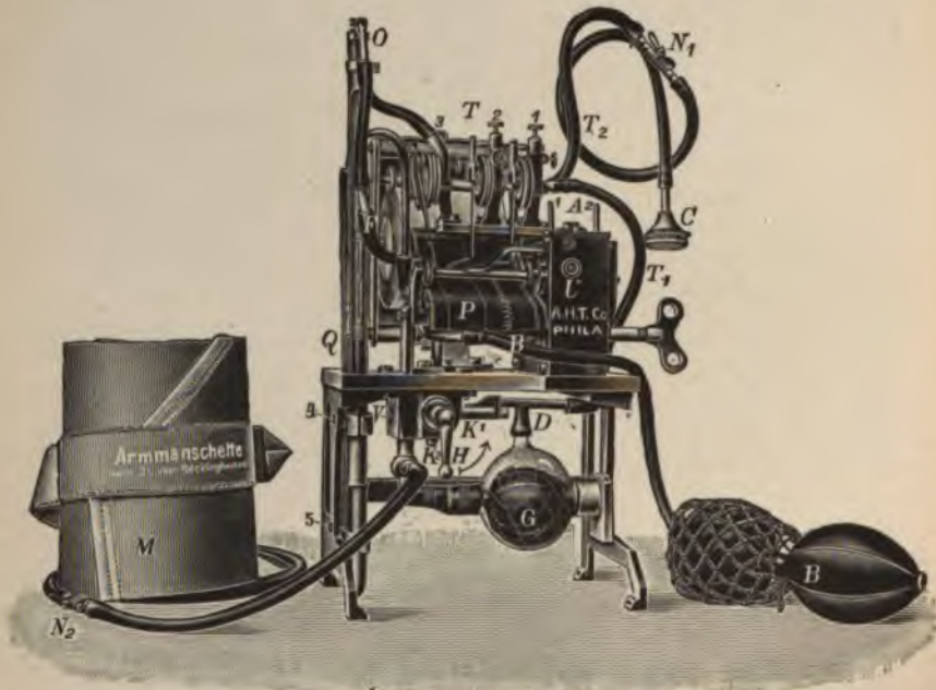
FIG. 40.—The Uskoff sphygmotonomograph.
