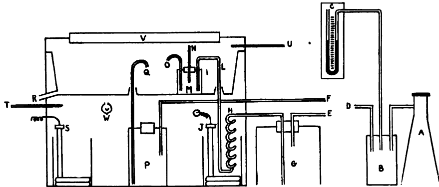
FIG. 3.—Injection apparatus.
