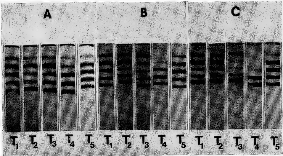
Fig. 3.- Separación electroforética de las isoenzimas de LDH de macerados de cerebro de A. olivaceus en geles de poliacrilamida al 7% almacenados a distintas temperaturas, T 1 - T 5 : + 49C, 09C, -49C, -309C, -1809C. A, B y C: 2,8 y 16 días. Los geles fueron cargados con 50 ug. de proteínas.
