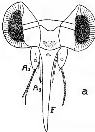
Fig. 5a. Zoëa cabeza de adelante. A 1 y A 2 antenas 1 y 2. F. espina frontal.
