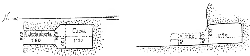
Fig. 2. a —Cueva d'en Ruyra. (Planta y sección.)
