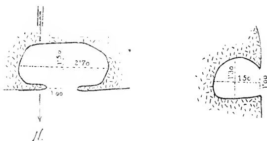
Fig. 4.ª—Cueva de Solius. (Planta y sección.)
