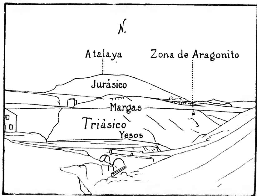
Situación del yacimiento de aragonitos enclavado en la margen derecha del Arroyo del Chorrillo, extramuros de Cabra.
