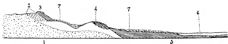
Relaciones entre los materiales de Gran Canaria, según Calderón. 1. Traquita; 2. Fonolita; 3. Tefrita; 4. Andesita augítica; 5. Basalto feldespático; 6. Formación terciaria; 7. Aluviones.
