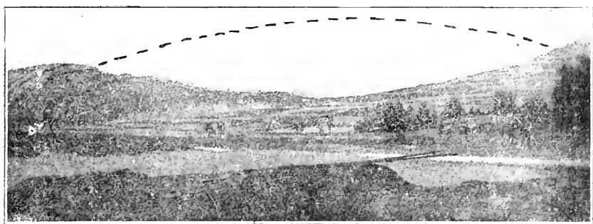
Anticlinal del Neocomiense en Portarubio, provincia de Teruel.
