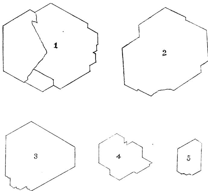
Fig. 1. a .—Secciones de berilos de Pontevedra. 1, Coutadas (Viascon); 2, Cabanelas (Viascon); 3, Sotomayor (Mos); 4, Campo d'Armida (Cerpozones); 5, Tres Hermanas (Pontevedra). (Todas a su tamaño.)
