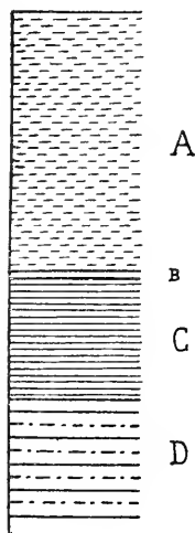
Fig. 2. a —Corte del pozo sin revestir en la finca del Sr. Christias. A, Porción superior de la tierra negra, degenerada en la superficie (2 metros).—B, Capa de sulfatos terciarios.—C, Porción inferior de la tierra negra (1 metro).—D, Margas azules sarmatienses. Escala de 1 : 50.
