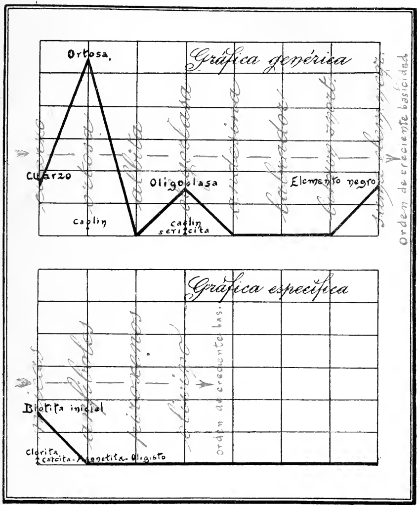
Representación gráfica de la composición mineralógica de una Siemite micacea de Gieringer Loch, Peterstal, Schwarzwald. Colección Rosenbusch, núm. 30.
