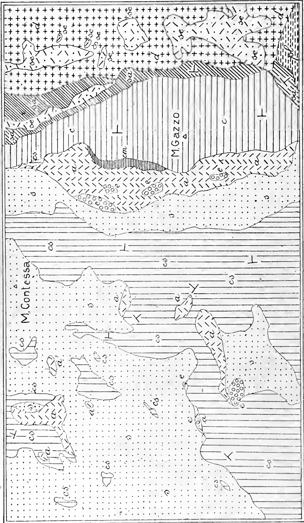
Fig. 13. — Serie Mesozoica: c . calcare dolomitico; cm . scisti calcarei argillosi; cs . calcescisti; s . serpentina; e . eufotidi; a . anfobliti. — Serie Eocenica: sa . scisti calcarei argillosi; d . diabase; se . serpentina; — pl . marne pioceniche. (1:25.000).
