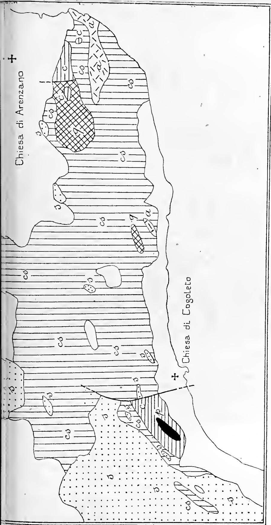
Fig. 9. — p. scisti rasati (permiano?); c. calcare dolomitico (trias medio); q. quarziti (trias inf.); cs. calcescisti mesozoici; a. amfiboliti e cloritescisti; s. serpentine e peridotiti. Le parti in bianco sono occupate da terreni neogenici. (1:25.000).
