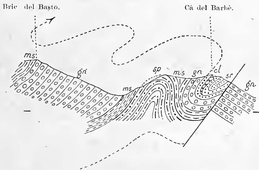
Fig. 1. — ms. micascisti; gn. gneiss; msg. micascisti quarziticci; as. anfiboliti; sp. scisti plumbei; cl. calcarei a lastre; sr. scisti rasati. (1:25.000).
