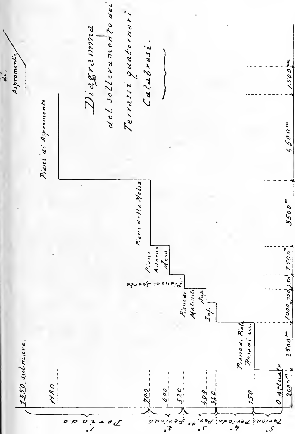
Fig. 2. La scala per le distanze è 1/10 di quella delle altezze.
