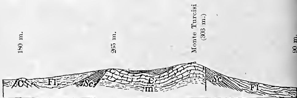
W.N.W. Fig. 5. — Sezione del Monte Turcisi nella scala di 1:25.000. E.S.E.
