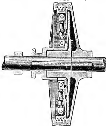
Friktionskoppling.
