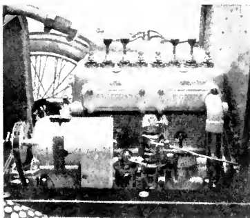
T. v. Fyrcylindrig automobilmotor med förgasaren och dynamon. T. h. Växellådan till cardandrivna automobil.
