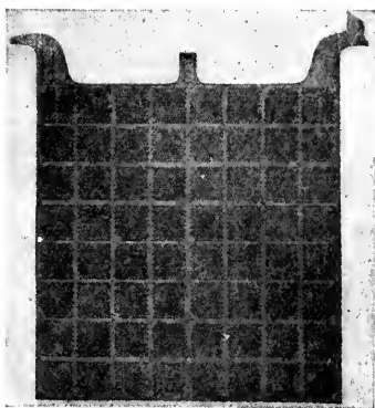
Negativ platta till blyackumulator.
