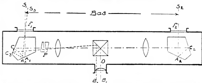
Fig. 1. Schematisk bild av Barr and Stroud's avståndsmätningssinstrument.
