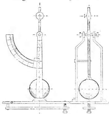
Pendelanemometer.
