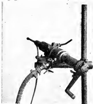
"Dux" borrhålsborrmaskin av Atlas' tillverkning.
