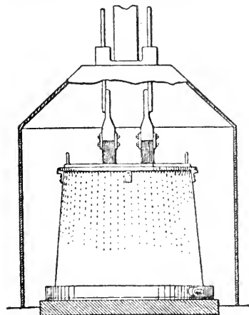
Elektrisk ugn för framställning av alundum.
