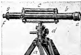
Avvägningsinstrument, tillverkat av Fr. J. Berg, Stockholm.
