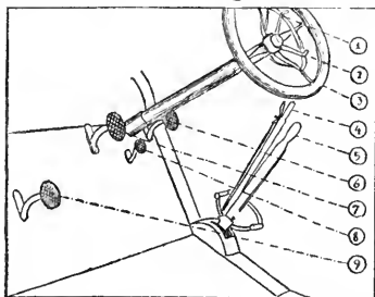
Styr- och regleringsanordningar å automobil. 1. Tändning. 2. Handgas. 3. Ratt. 4. Handbroms. 5. Växelspak. 6. Fotbroms. 7. Kona. 8. Fotgas. 9. Starter.
