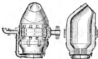
Fig. 3. Modern konverter.
