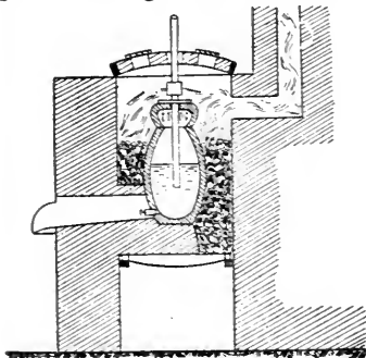
Fig. 1. Bessemers första ugn.
