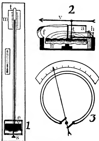
Barometrar.
