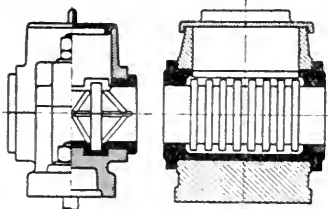
Två kamlager.
