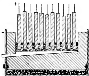
Halls elektriska aluminiumugn.
