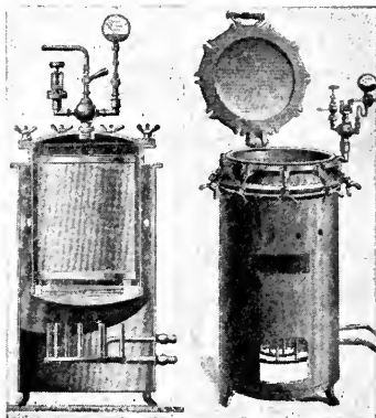
Autoklaver för laboratoriebruk. Uppvärmning med gaseldning.
