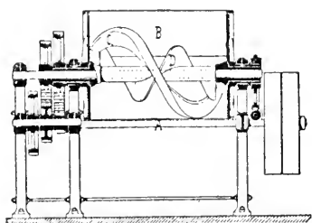
Fig. 2. Degknådningsmaskin.
