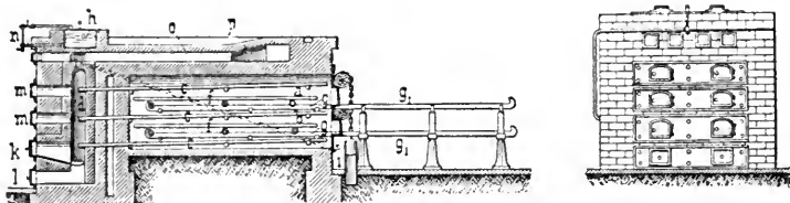
Fig. 4. Modern bakugn.
