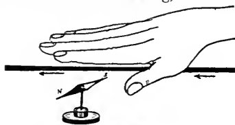
Ampères regel.
