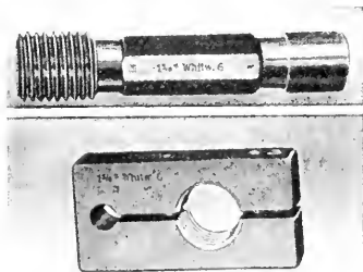
Gängtolkar för mutter (överst; kombinerad med cylindertolk) och skruv.
