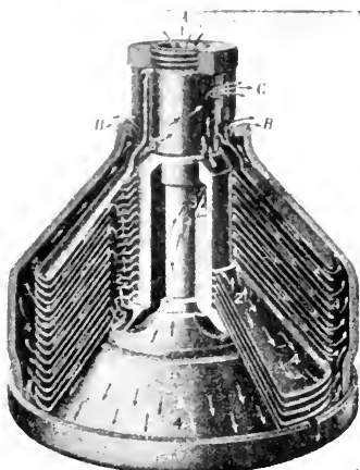
Alfa-insats i mjölksseparator. A Inlopp för mjölk, B utlopp för skummjolk, C utlopp för grädde (jfr vid. texten).
