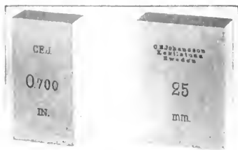
Passbitar ur kombinationsmåttsetsat. T. v. Mått i eng. tum. — T. h. i mm. Måtten innehållas i bitarnas bredd.
