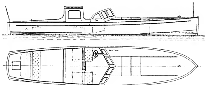
Motorbåt. Profil och plan av racermotorbåt. Längd 10 m., bredd 2,00 m., 120 HK:s motor, fart 26 knop.
