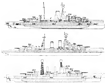
Sidopansarets utsträckning å slagskepp. "Resolution" (eng.), "Nagato" (jap.), "Maryland" (För. Stat.). (Siffrorna beteckna pansarets tjocklek.)
