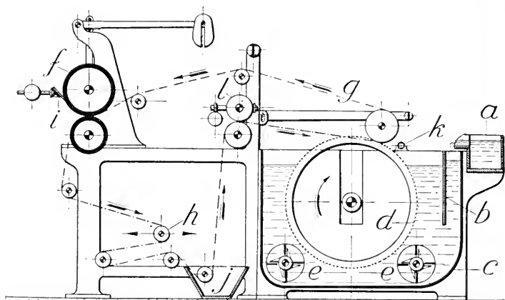
Arkupptagningsmaskin. a massarädda, b skumbräde, c massakar, d cylinder, e omrörare, f formatvals, g filtt, h spännvals, i schaber, j filttvätt, k spritsrör, l filtpress.
