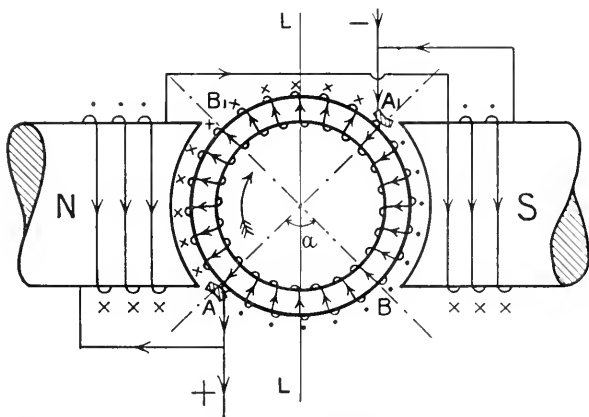
Motmagnetisering. Linjen L—L utvisar det magnetiska neutralläget. \alpha = dubbla borstförskjutningsvinkeln.
