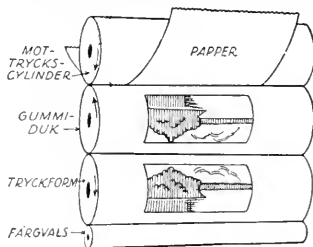
Schematisk bild av offsetpress.
