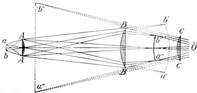
Strålgången i ett mikroskop. AA objektiv, BB okularets kollektivlins, CC dess ögonlins. Ö öga. ab föremål. a'b' dess avbildning genom objektivet, a''b'' genom objektiv och kollektivlins, a'''b''' den på avståndet för tydligt seende tänkta jämförelsebild.
