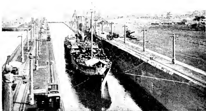
Panamakanalen. Gatförlussarna. Fartyget bogseras av elektriska traktorer.
