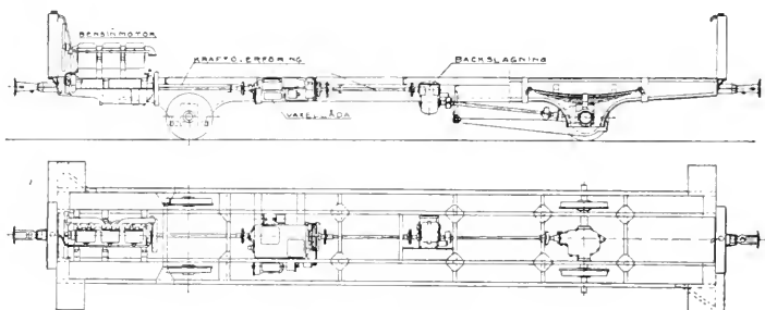
Underrede och maskineri till smalspärig bensinmotorvagn.
