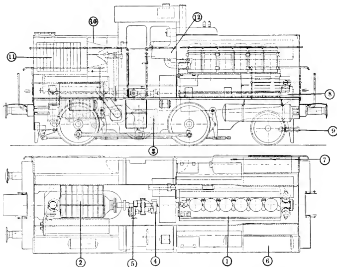
Dieselmotorlokomotiv med Lentzöverföring. 1. Dieselmotor (250 HK). 2. Oljepump ("avsändare"). 3. Drivmotor ("mottagare"). 4. Belysningsmaskin. 5. Kylvattenpump. 6. Behållare för bromsluft. 7. Behållare för startluft till dieselmotorn. 8. Kompressor för bromsluft. 9. Mellankylare till kompressorerna. 10. Fläkt. 11. Vattenkylare. 12. Ljuddämpare.
