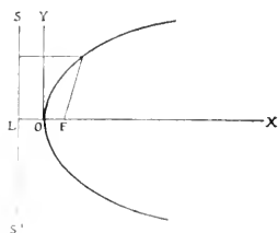
Parabel.
