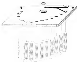
Regleringsmotstånd, schematisk teckning. Endast de främre motståndsspirlarna äro utritade.
