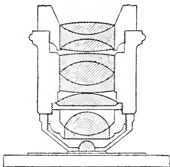
Mikroskopobjektiv för oljeimmersion.
