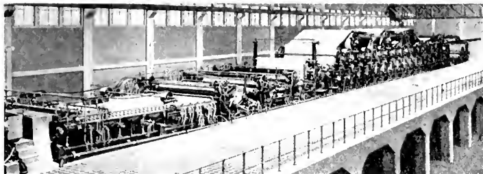
Fourdriniermaskin (virapartiet närmast).
