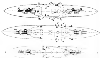
Artilleriets uppställning å slagskepp. "Resolution" (eng.), "Nagato" (jap.), "Maryland" (För. Stat.). (Siffrorna beteckna kaliber.)
