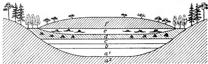
Mosse. Schematisk teckning av lagerföljden. a 1 gyttja, a 2 torvmarkens underlag (berg, sand l. lera), b dy, c starrtorv, d alkärrtorv, e tallmosstorv, f vitmosstorv.
