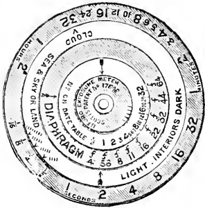
Fig. 176.—ILFORD EXPOSURE METER
