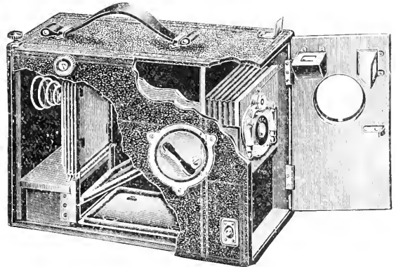
Fig. 671.—“DAI CORNEX.”
