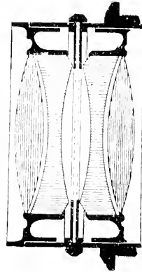
Fig. 525.—UNOFOCAL LENS.
