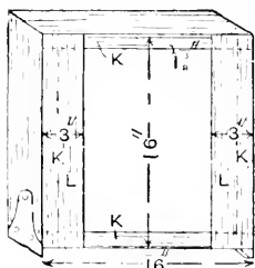
Fig. 55.— SLIDING FRAME.
