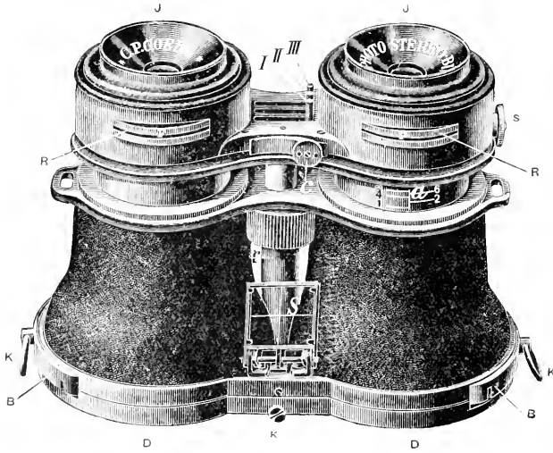
Fig. 664.—GOERZ STEREO BINOCULAR.
