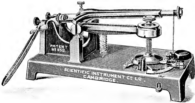
Fig. 722.—ROCKING MICROTOME.
