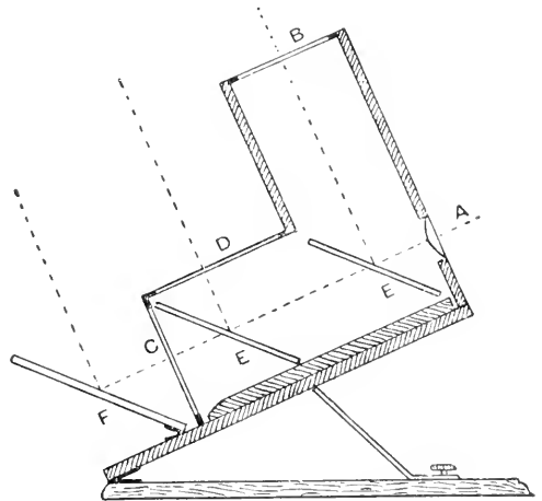
Fig. 576.—THE IVES KROM-KOP.
