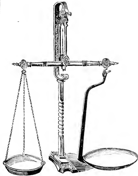
Fig. 128.—SCALES.
