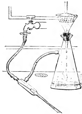
Fig. 138.—FILTER PUMP.
