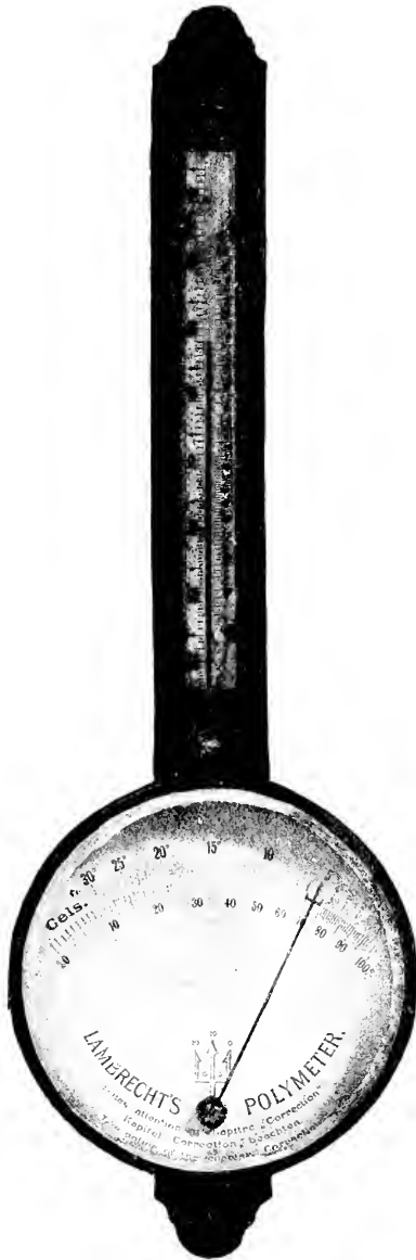
Fig. 303.—HYGROMETER.
