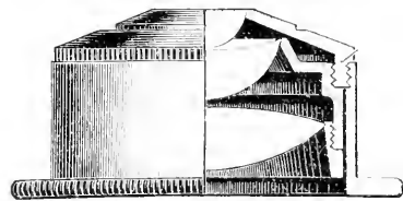
Fig. 705.—ABBE CONDENSER. (NUMERICAL APERTURE 1.4.)
