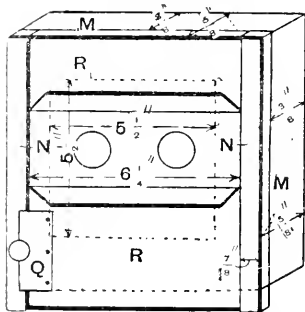
Fig. 81.—FRONTBOARD FRAME.
