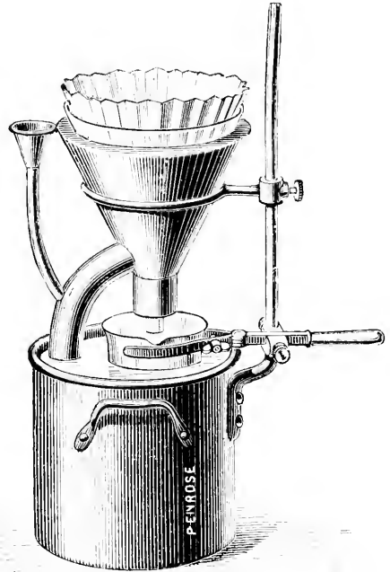
Fig. 884.—WATER-BATH FILTRATION APPARATUS.
