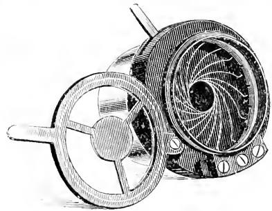
Fig. 712.—CENTRE STOP.
