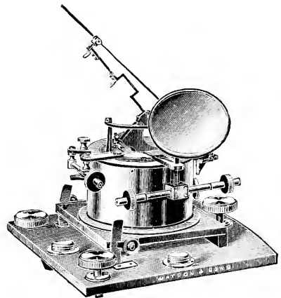
Fig. 675.—HELIOSTAT.
