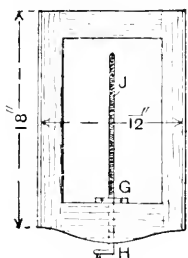
Fig. 54.— EXTENSION FRAME.
