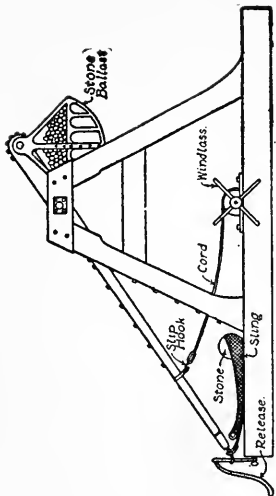
FIG. 228. — A Trebuchet.
