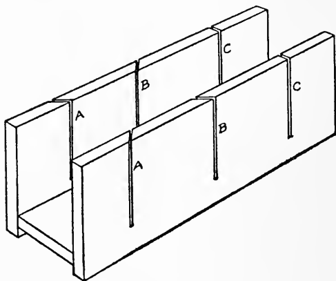
FIG. 12. — A Mitre-box.
