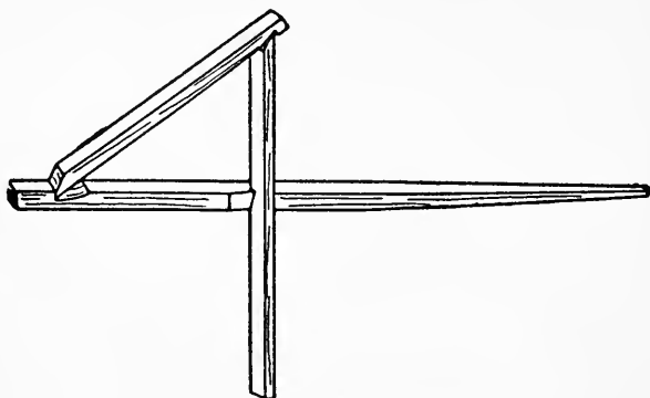
FIG. 215.—The Figure-four.
