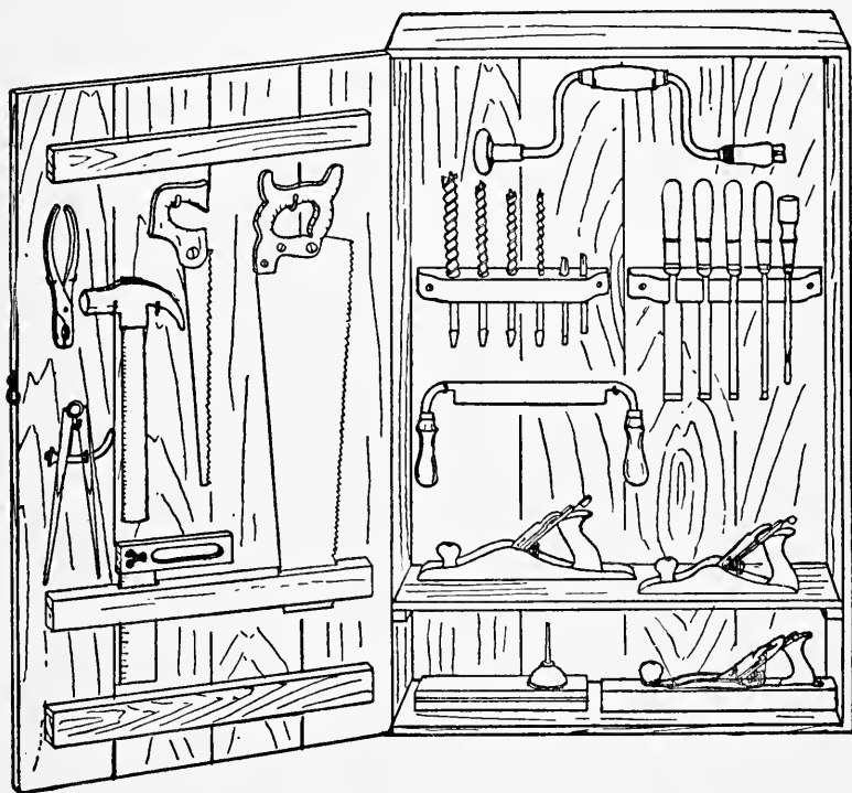
FIG. 15.—Tool-cabinet.
