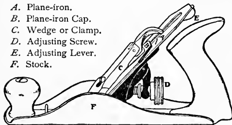
FIG. 24. — Stanley Iron Plane.
