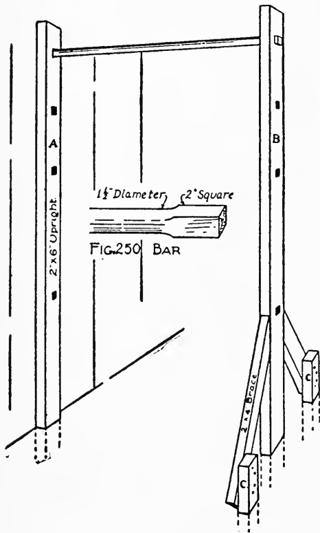
FIG. 251. — The Horizontal Bar.
