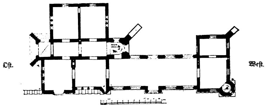
26. Grundriß von Williamscastle (Richmond).
