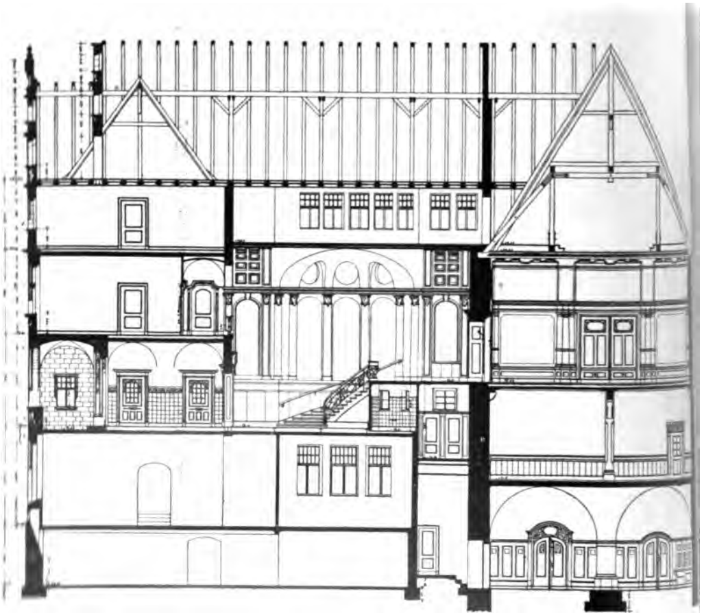
Querschnitt des geplanten Neubaus.
