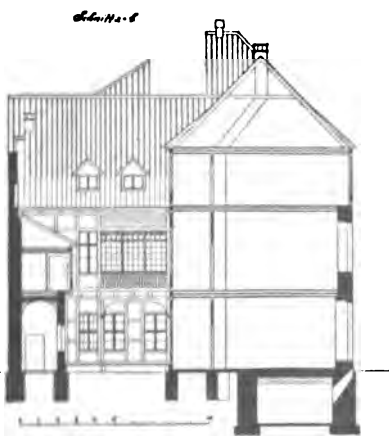
13. Querburchschnitt der städtischen Münze.
