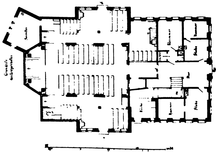
2 a. Grundriß des Erdgeschosses der St. Nicolaikirche.
