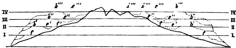
Schematischer Durchschnitt einer Insel mit Riffen.
