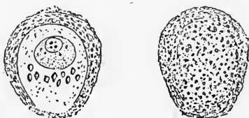
FIG. 154.— Pseudodifflugia archeri . \times 200 .
