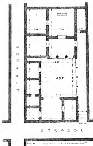
Hausgrundriß von Priene (nach Wiegand und Schrader, Priene)
