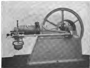
Fig. 17. Ottoscher Gasmotor.
