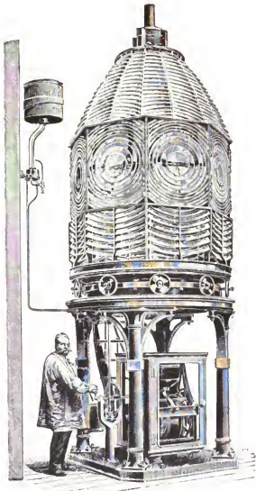
Fig. 4. Fresnel-Apparat erster Ordnung.
