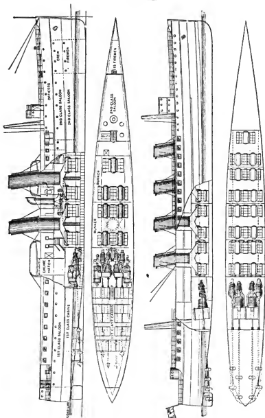
Fig. 16. Zwei Feuerlöcher Kanalampfer.
