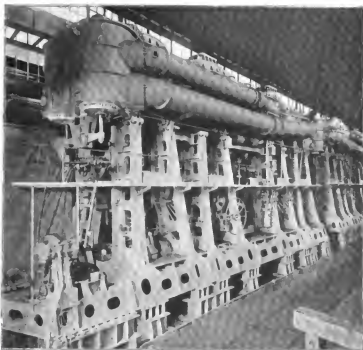
Fig. 11. Betriebsmaschine des Dampfers „Deutschland“ von 33000 Pferdestärken.
