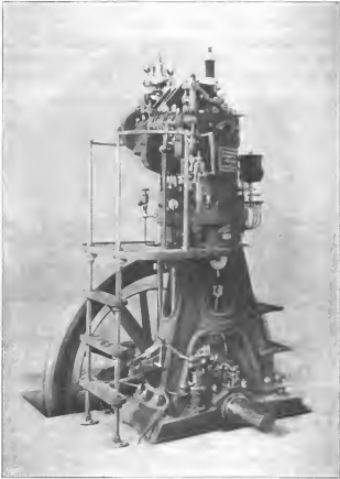
Fig. 20. 25pferdiger Dieselscher Warmemotor.
