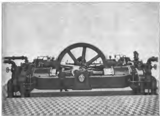
Fig. 19. 600pferdige Deutscher Gaskraftmaschine.
