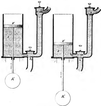
Fig. 5. Wasserschraubenmaschine.
