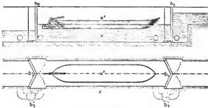
Fig. 4. Kammerschleuse.
