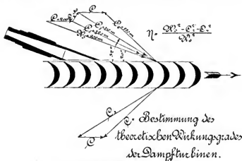
Fig. 14. Schaufelung und Dampf Düse zum Lavalrad.
