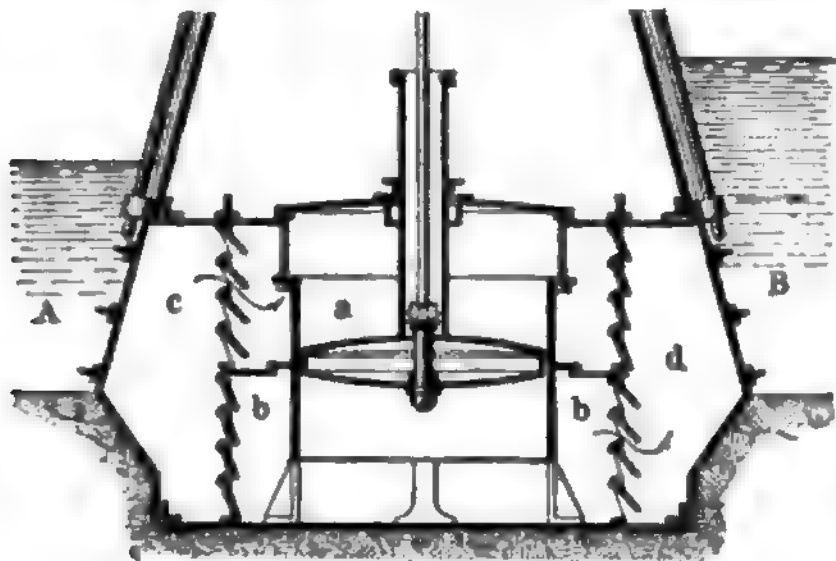
Fig. 9. Fijnjesche Kastenpumpe.
