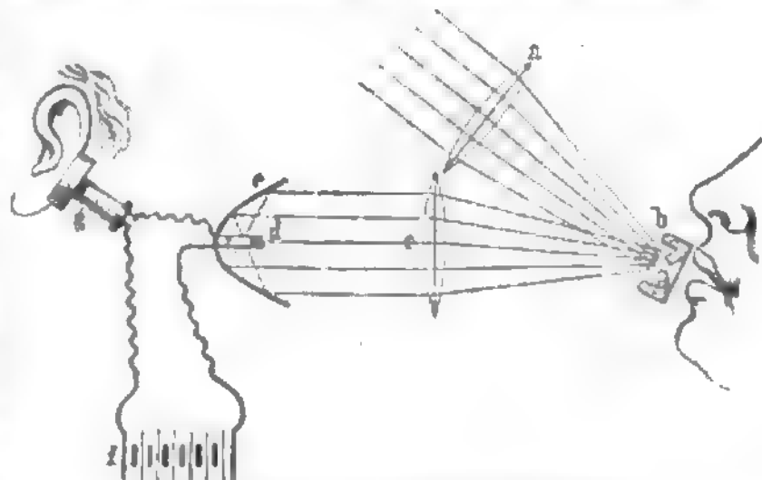
Bells Photophon (schematische Darstellung).
