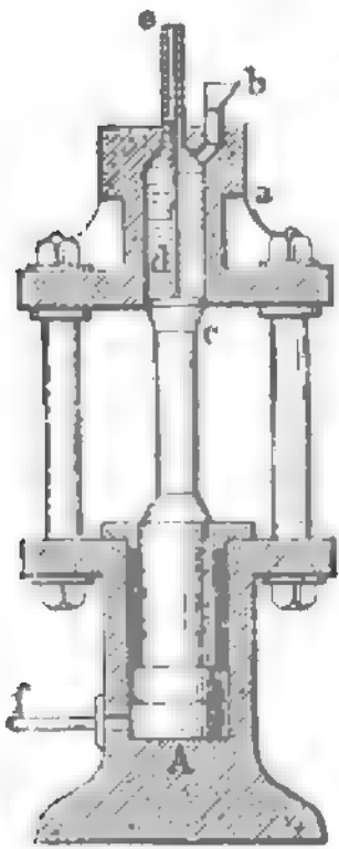
Fig. 2. Röhren- presse.
