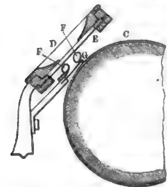
Fig. 2. Zeichengegebender Apparat des Phonographen.
