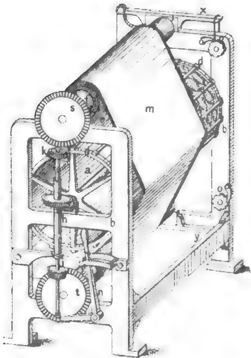
Rauhmaschine.
