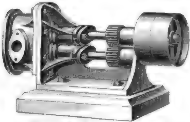
Fig. 20. Rotationspumpe, Ansicht.
