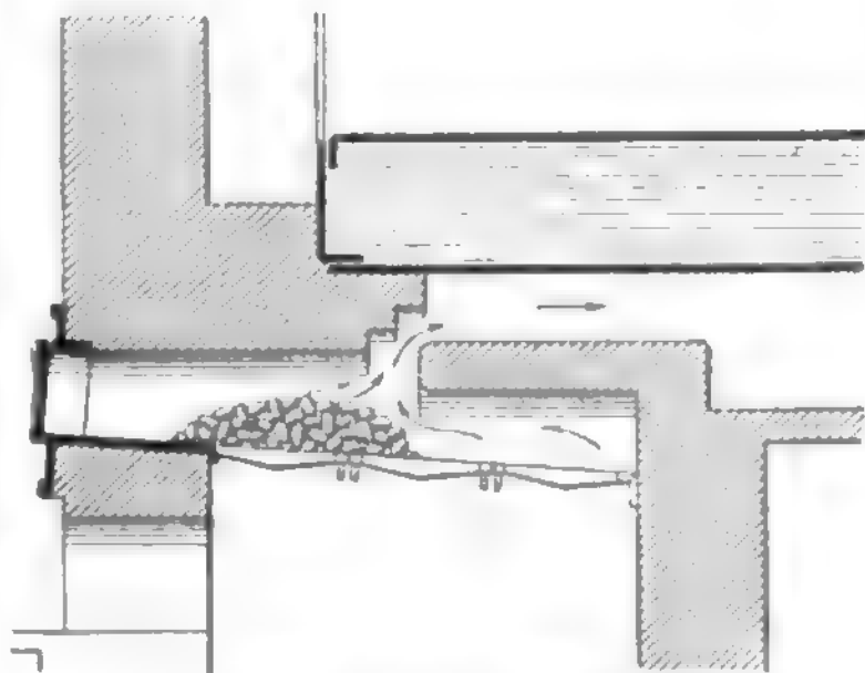
Fig. 5. Adams Feuerung.
