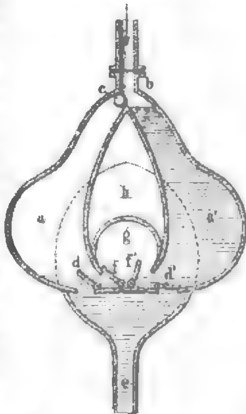
Fig. 1. Schematische Darstellung des Pulsometers.
