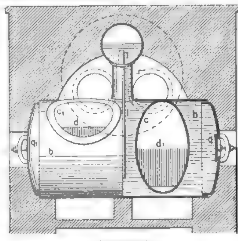
Fig. 6 u. 7. Ten-Brinksche Feuerung.
