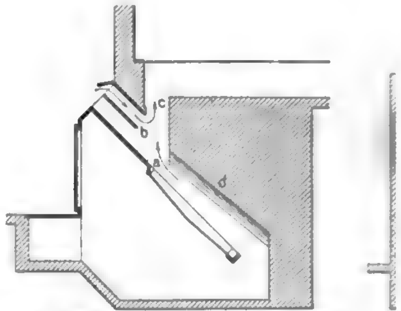
Fig. 8. Abgeänderte Ten-Brinksche Feuerung.
