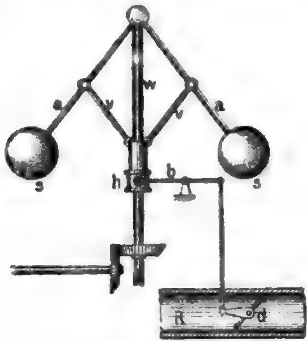
Fig. 1. Regulator mit direkter Übertragung.
