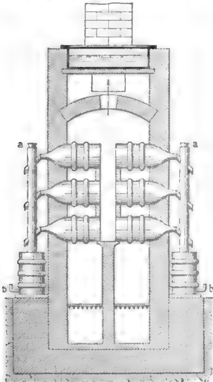
Ofen zur Destillation des Phosphors.
