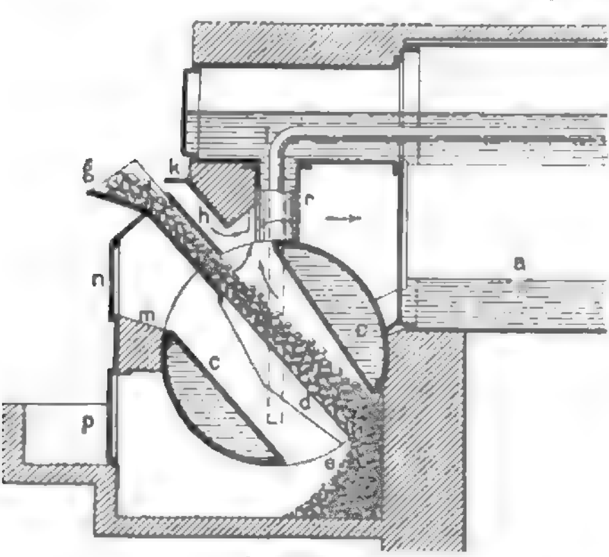
Fig. 6 u. 7. Ten-Brinksche Feuerung.
