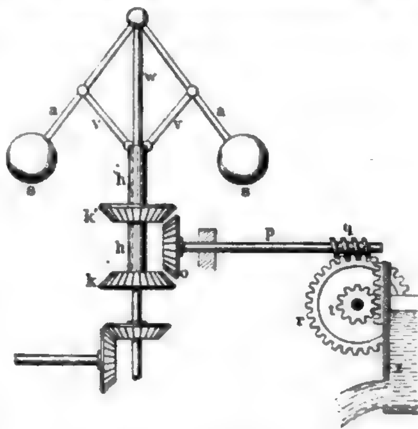
Fig. 2. Regulator mit indirekter Übertragung.
