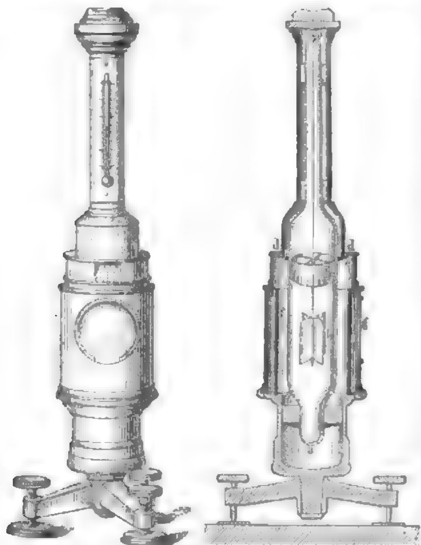
Fig. 6. Galvanometer.
