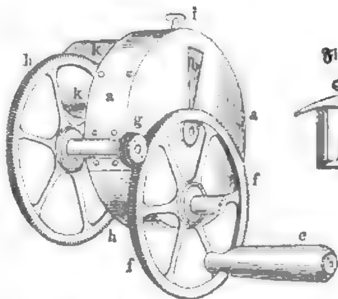
Fig. 1-3. Phosphoroskop.
