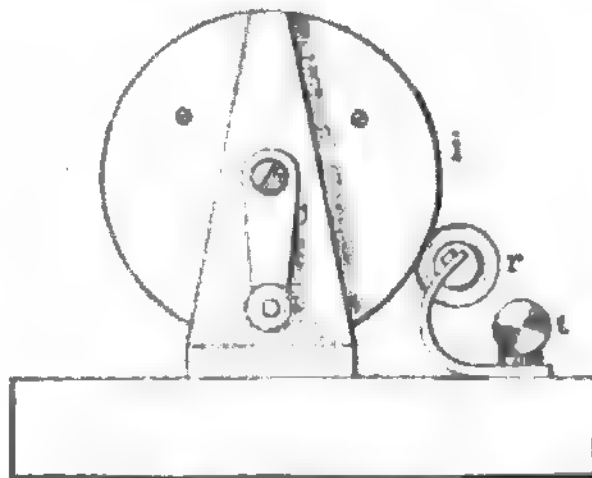
Fig. 2 Vorderansicht.
