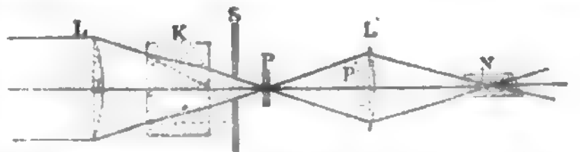
Einrichtung des Polarisationsapparats von Duboscq.
