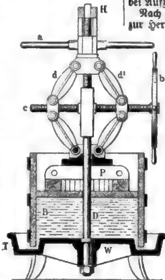
Fig. 1. Kniehebelpresse.
