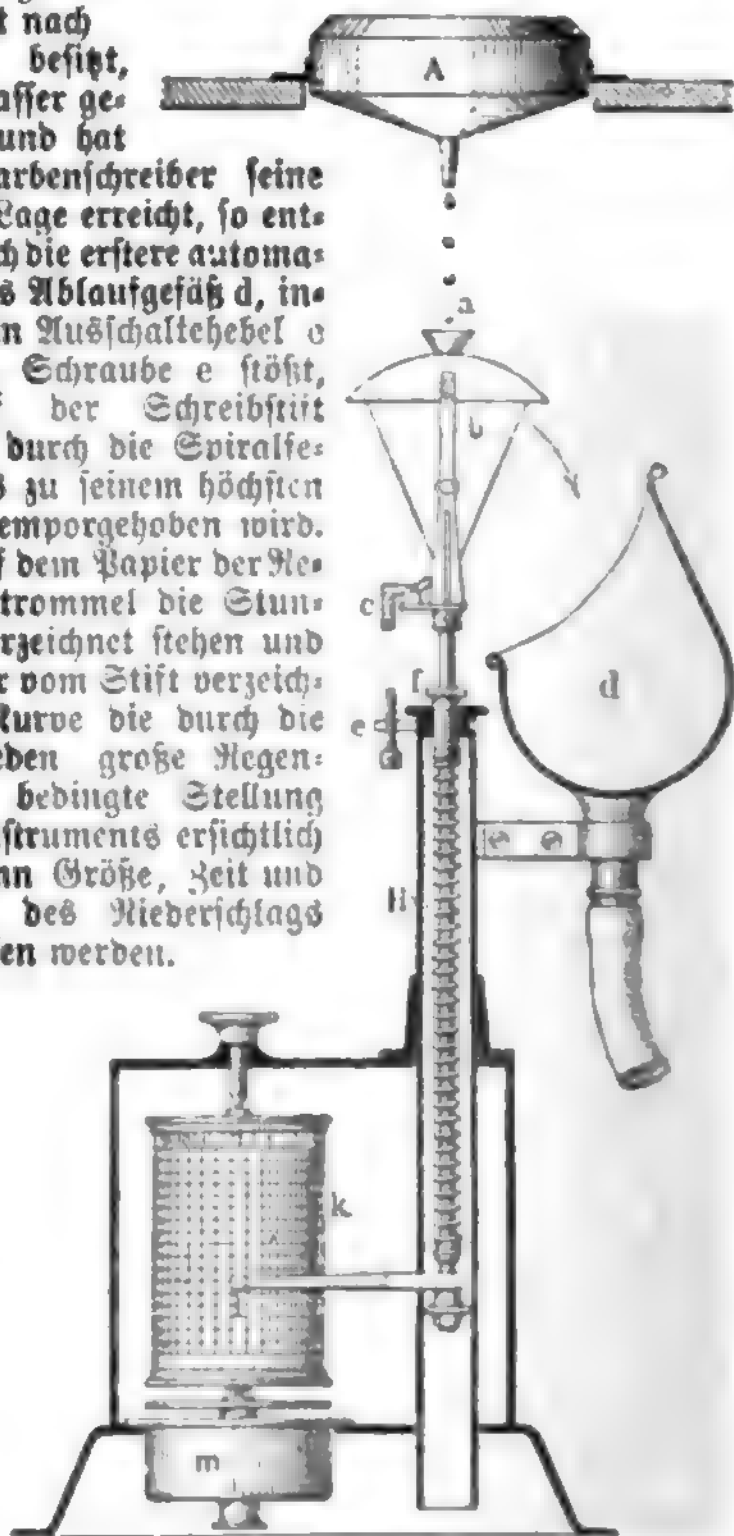
Gottingers selbstregistrierender Regenmesser.
