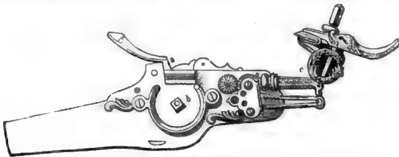
Radschloß.
