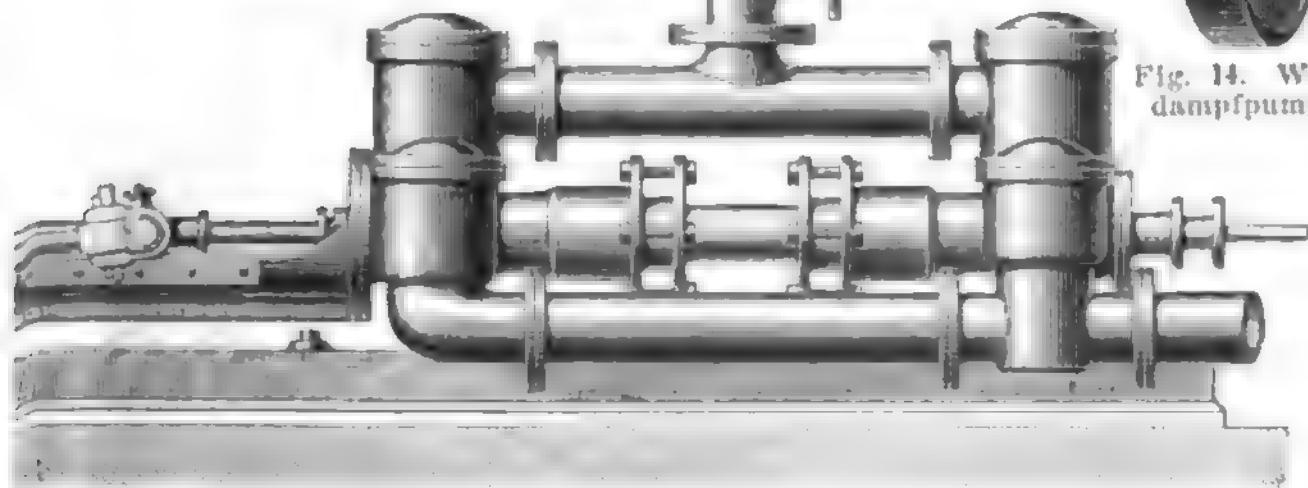
Liegende doppelt wirkende Schachtpumpe.
