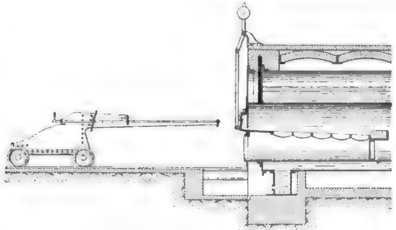
Fig. 11. Struplers Kohlenaufschütter auf Lafette.
