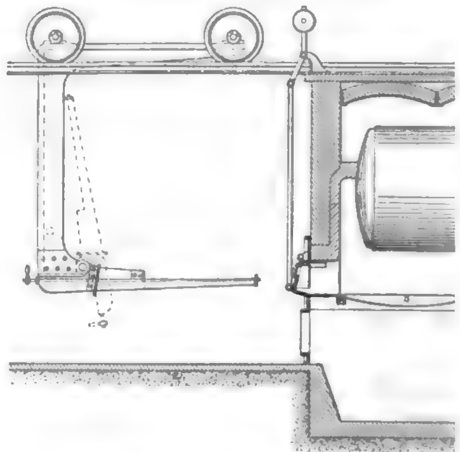
Fig. 12. Struplers Kohlenaufschütter, hänge
