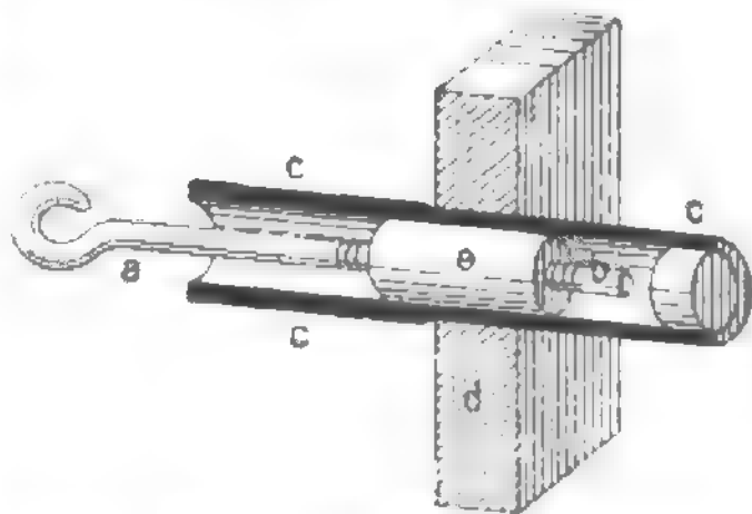
Fig. 1. Rührer Dorn.
