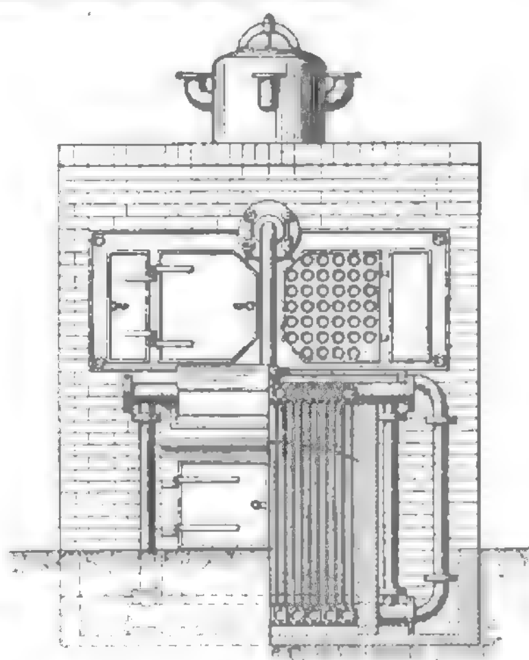
Vorderansicht.
