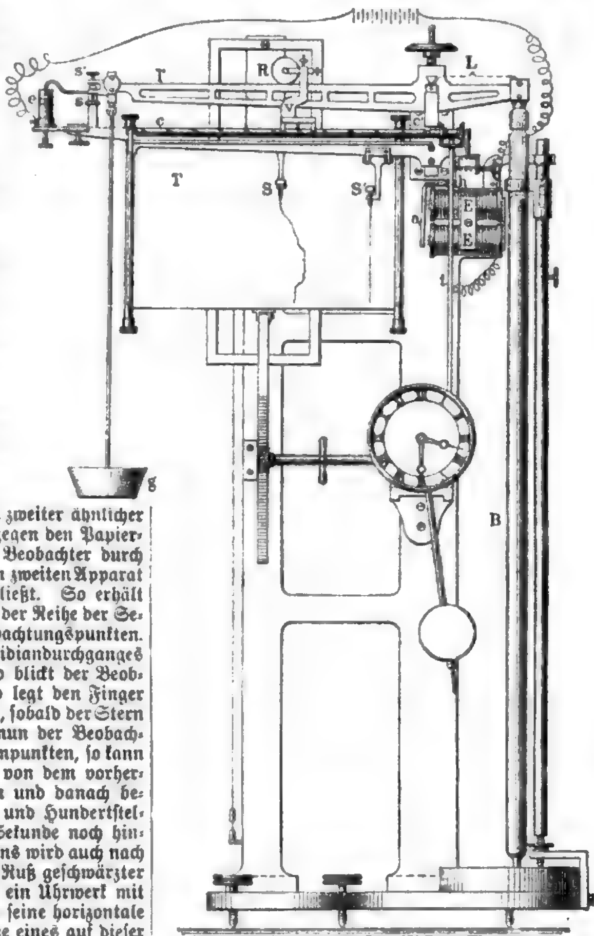
Fig. 1. Wagebarograph von Fuch-Sprung.
