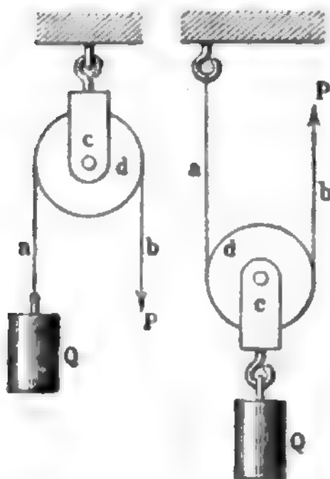
Fig. 1. Feste Rolle. Fig. 2. Lose Rolle.
