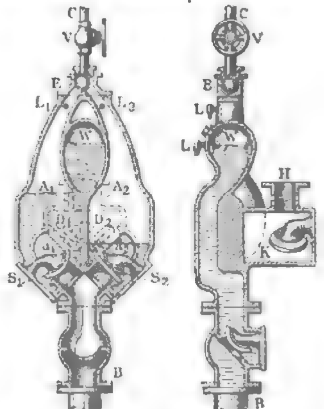
Fig. 2 u. 3. Hall'sches Pulsometer in Längs- und Querschnitt.
