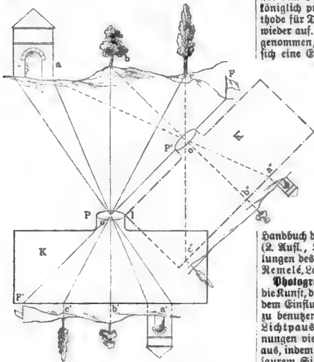
Photogrammetrie.
