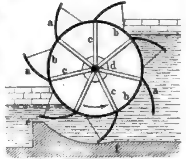
Pumprad.
