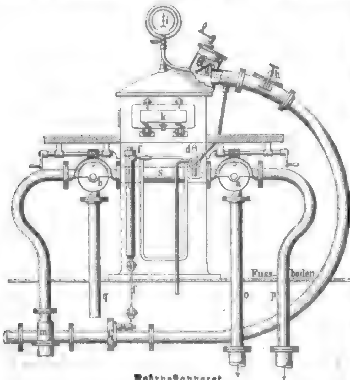
Rohrpostapparat.
