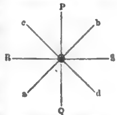
Fig. 13. Zerlegung der Schwingungen.
