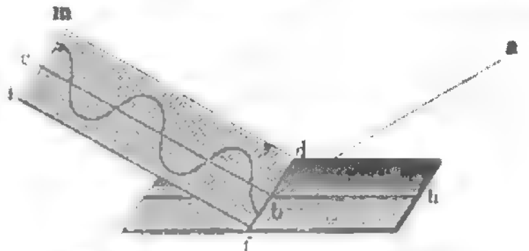
Fig. 8. Polarisation durch Reflexion.
