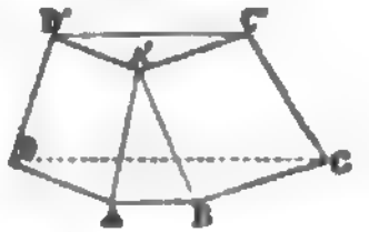
Fig. 1 u. 2 Prismatoide.
