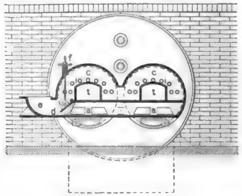
Vorderansicht.
