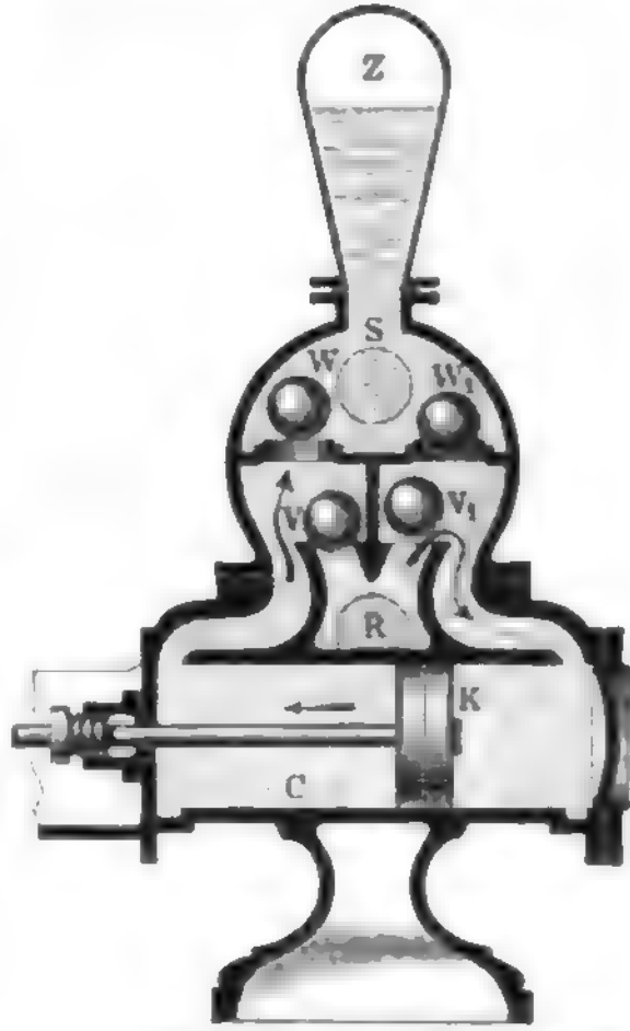
Fig. 6. Liegende Pumpe mit Druckwindkessel.
