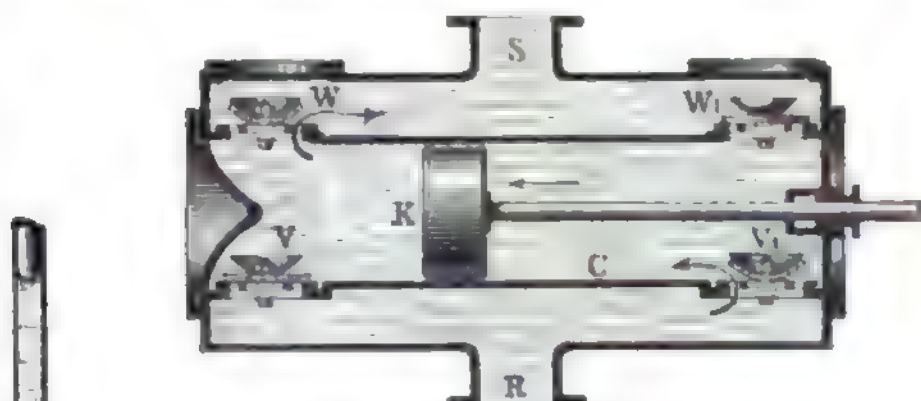
Fig. 4. Liegende doppelt wirkende Pumpe.
