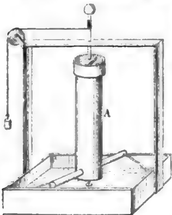
Eggerss Reaktionsrad.
