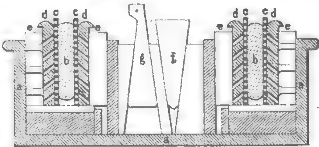
Fig. 3. Keilpresse.
