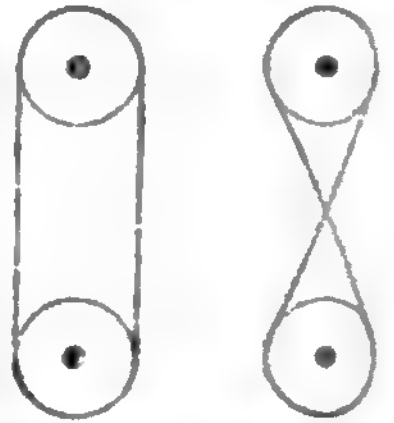
Fig. 1. Offener Riementrieb. Fig. 2. Gekreuzter Riementrieb.
