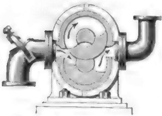
Fig. 21. Rotationspumpe, Querschnitt.
