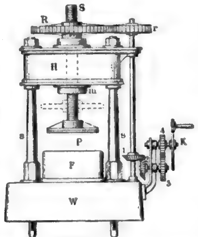
Fig. 2. Schraubendresse.
