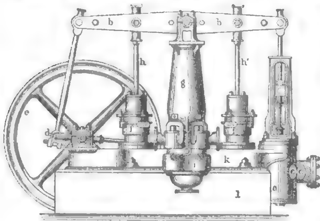
Fig. 15. Balancierdampfpumpe.
