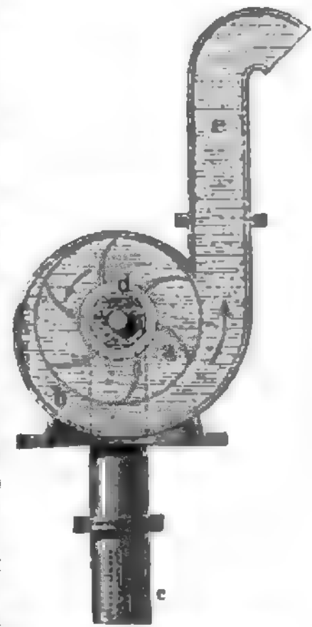
Fig. 22. Zentrifugalpumpe.
