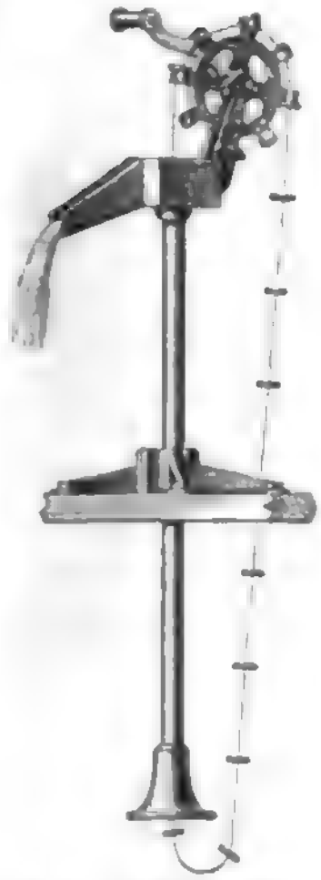
Fig. 11. Jauchepumpe.
