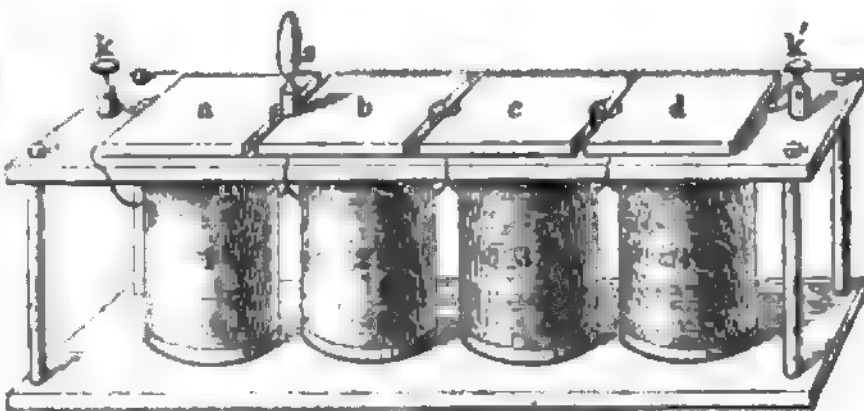
Fig. 3 Stöpselrheostat nach Siemens.
