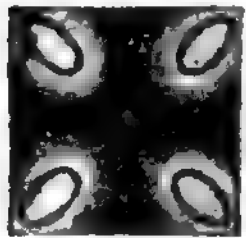
Fig. 17. Farbenerscheinung in gekühltem Glas.
