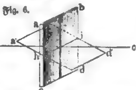
Fig. 5 u. 6. Versuch zur Ermittlung der Schwingungsrichtung.
