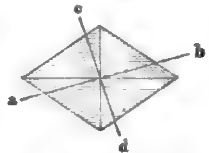
Fig. 12. Gipsblättchen.
