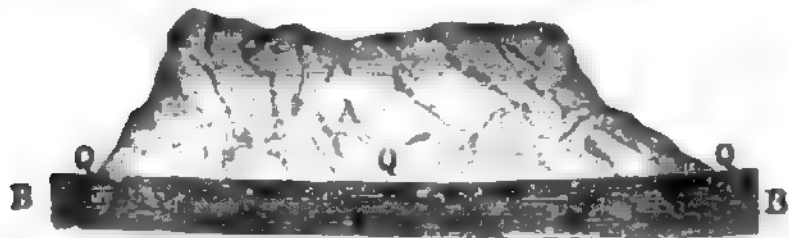
Fig. 1. Quellenbildung bei horizontaler wassersperrender Schicht.
