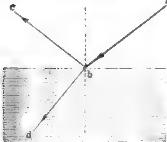
Fig. 11. Polarisationwinkel (Brewsters Gesetz).
