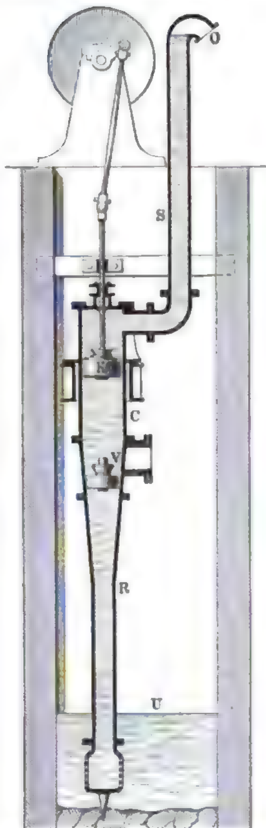
Fig. 1. Hubpumpe mit Steigrohr.
