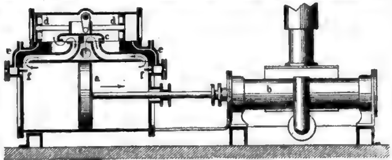
Fig. 20. Tangen-Pumpe.
