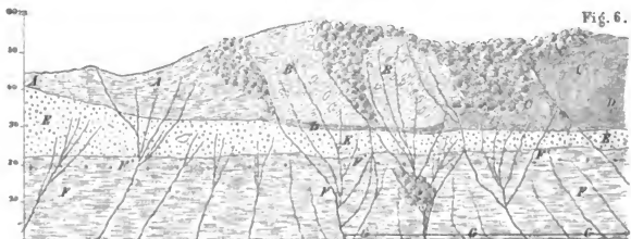
Ansicht der Puttenhamer Innleithe unterhalb Wasserburg.
