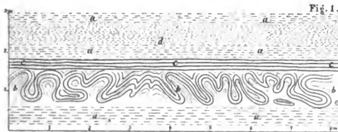
Schichtenstörungen im Bänderthon bei Vomperbach. 1:100.
