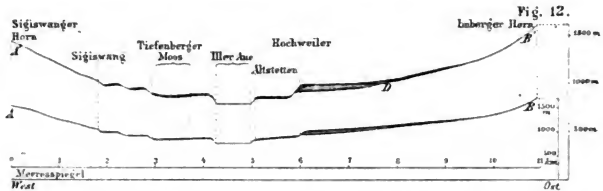
Querprofil des Illerthales oberhalb Sonthofen.
