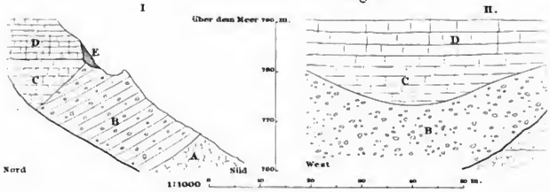
Profil am oberen Ende des Weiherburger Grabens bei Inns I von der Seite, II von vorn.
