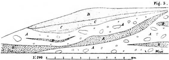
Schottergrube nördlich Starnberg.
