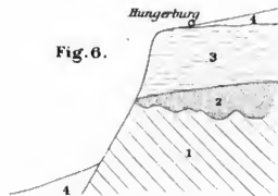
ca. 1:5000 Profil an der Hungerburg bei Innsbruck Copienach Pichler, Beiträge zur Geognosie Tirols Taf. I, Fig. VI. 1 Oberer Alpenkalk 2 Sand und Letten (Grundmoräne) 3 Tertiärconglomerat (Rother Breccie) 4 Diluvium (Schotter)
