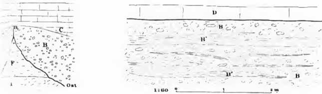
Grenze zwischen rother Breccie und Grundmoräne. bei a Fig. 1, II.
