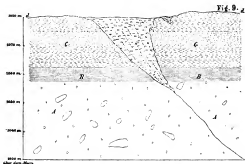
Südgehänge der Schlucht bei Holzleithen.
