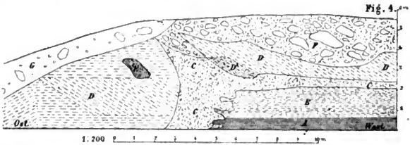
Schottergrube nördlich Starnberg.
