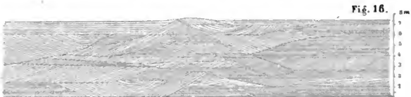
Struktur der diluvialen Nagelfluh. Grosshesselohe bei München.
