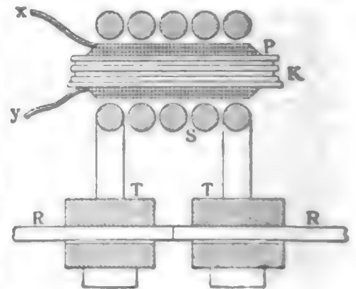
Fig. 2. Elektrischer Lötapparat.
