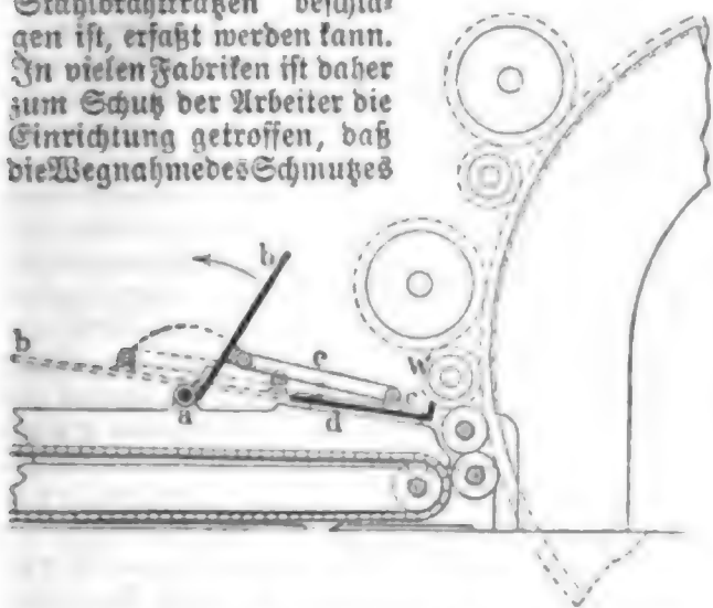
Fig. 3. Dietrichs Fangkorb für Walzenkrempel.
