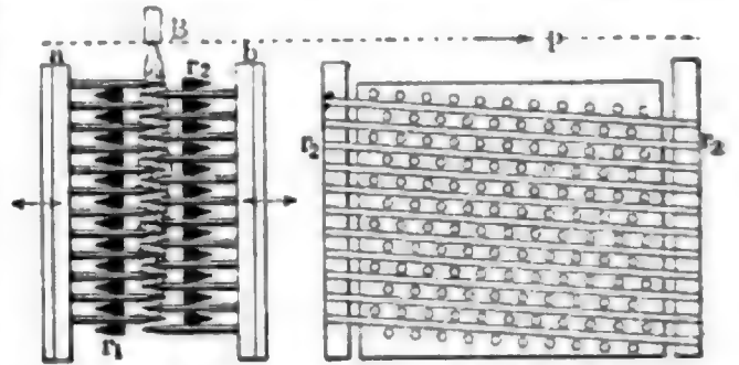
Fig. 1. Stechplatten.
