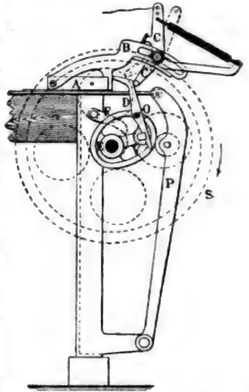
Fig. 4. Vorrichtung zum Vorsetzen der Lade.
