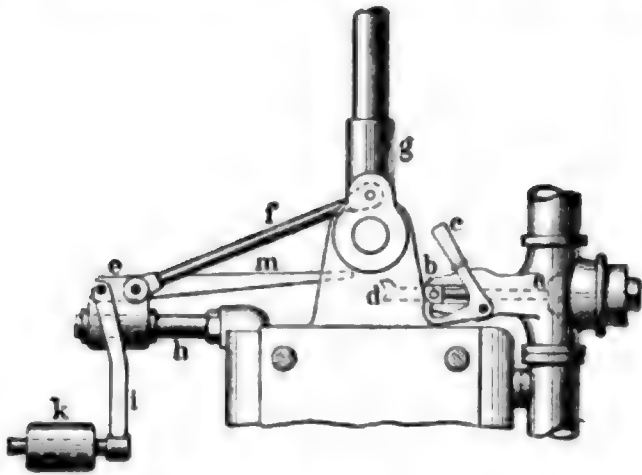
Fig. 3. Regulator zum Deutzer stehenden Motor.
