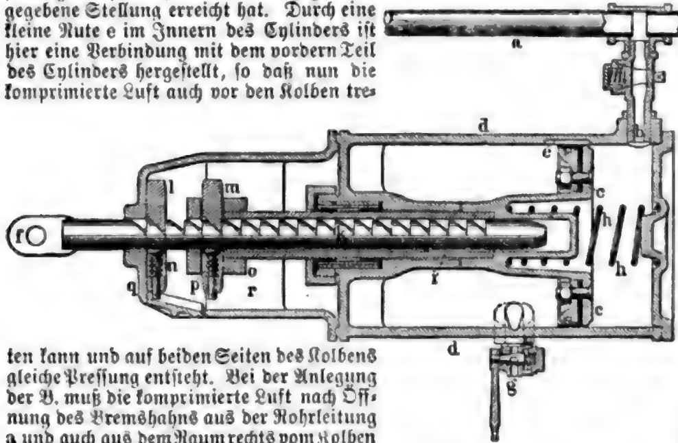
Fig. 1. Carpenterbremse.
