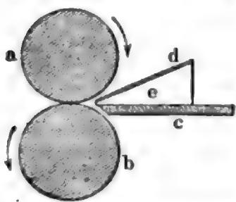
Fig. 3. Schutzvorrichtung von Satinierwalzen.
