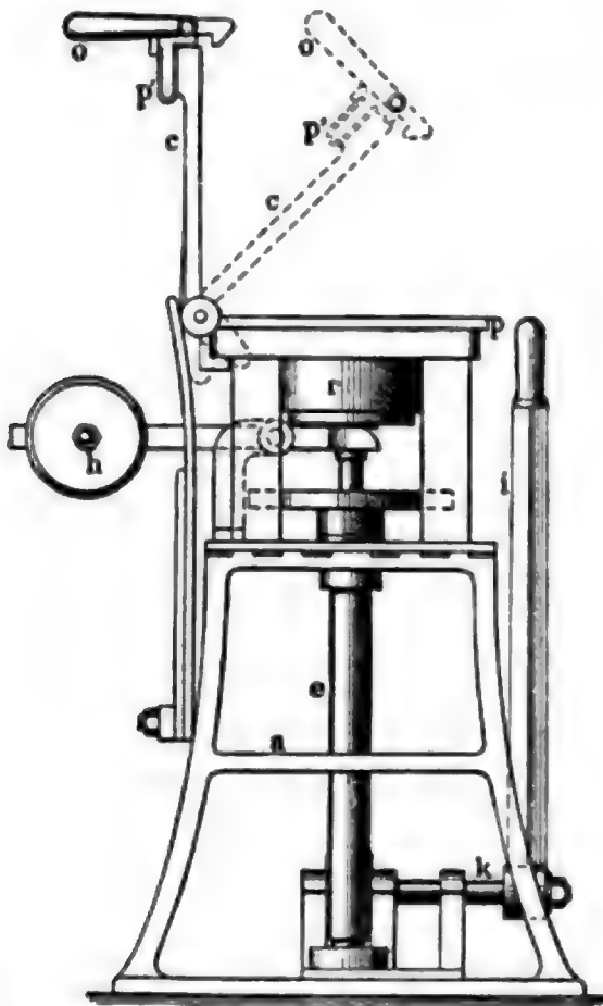
Fig. 4. Neue Teigteilmaschine von Brünig. Seitenansicht.
