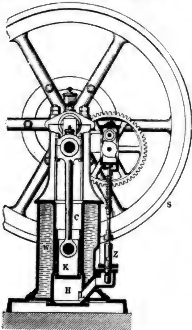
Fig. 1. Längsschnitt.
