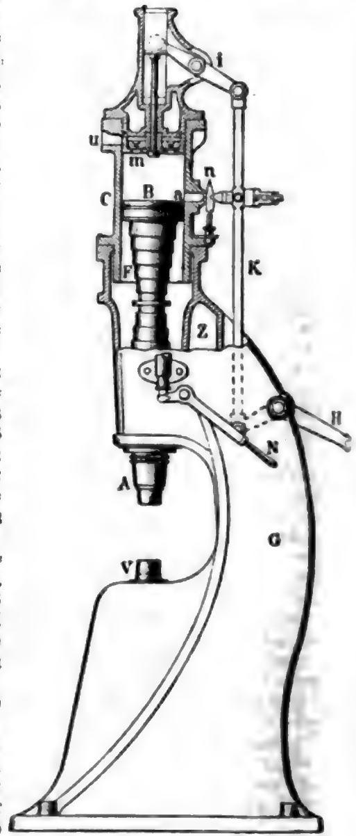
Fig. 2. Gashammer.
