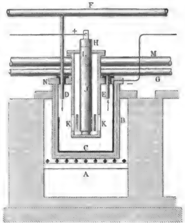
Fig. 1. Gräbel's Apparat zur Darstellung von Aluminium.
