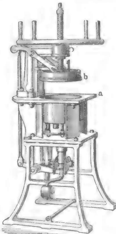
Fig. 2. Teigteilmaschine von Brüning.
