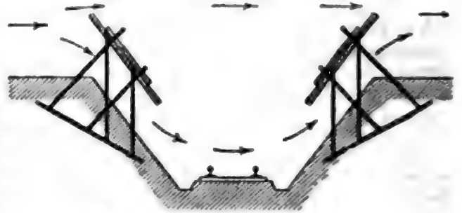
Fig. 3. Schneeschirm von Howie.
