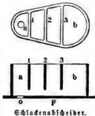
Schlackenabscheider.
