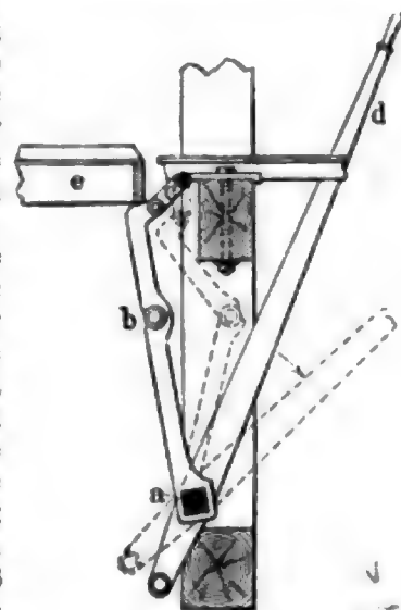
Fig. 3. Westmeyer'sche Schachtfalle.
