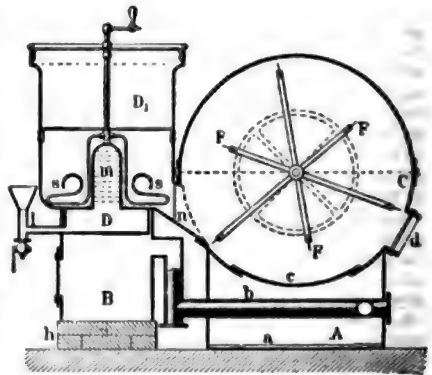
Federnreinigungsmaschine.
