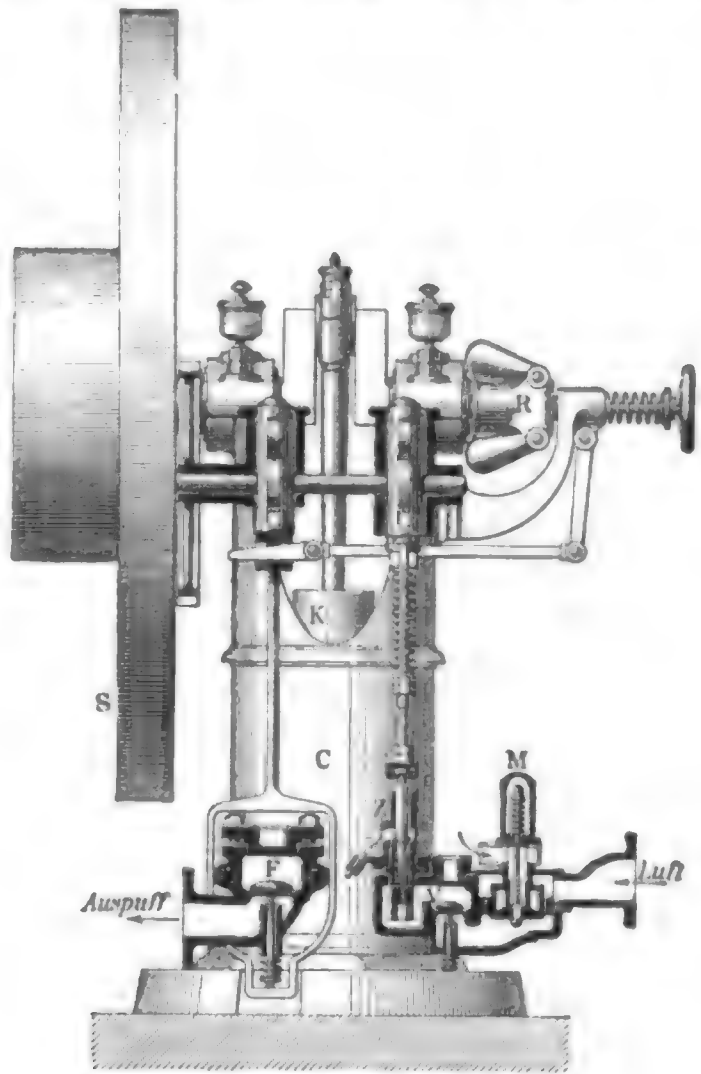
Fig. 2. Vorderansicht und Schnitt durch die Ventile
