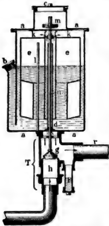
Fig. 4. Gasdruckregulator.
