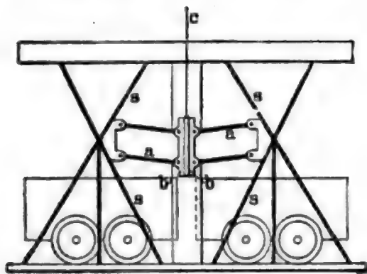
Fig. 2. Hoppsche Fallbremse.
