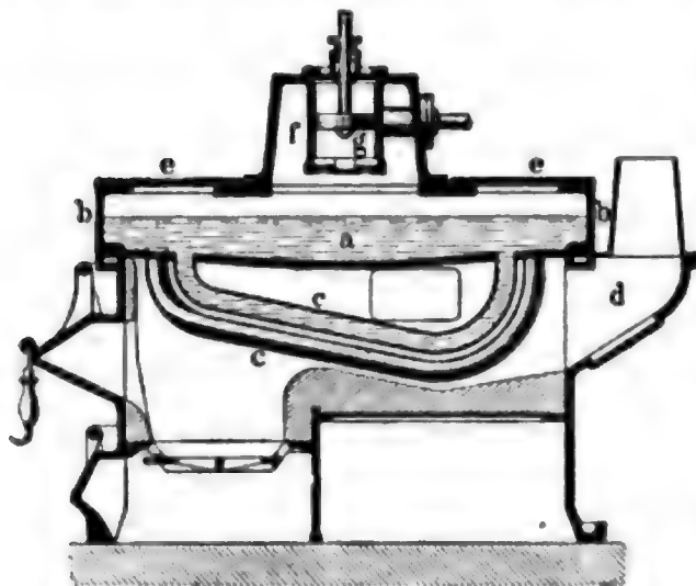
Kessel des Hoffmeister-Altman'schen Motors.
