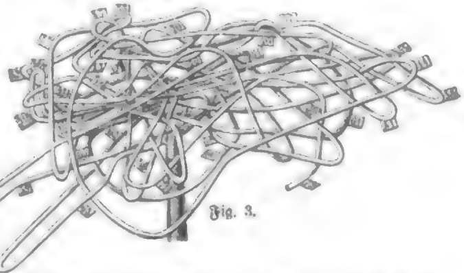
Fig. 1—3. Bewegung einer Erdpartikel während des Erdbebens zu Tokio, 15. Jan. 1887, dargestellt durch einen Kupferdraht nach den drei rechtwinkligen Komponenten des Erdbeben-diagramms. Die Zahlen geben die Sekunden an von 0—72. Nach S. Sekiya (viermalige Vergrößerung der vertikalen und horizontalen Bewegung).
