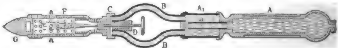
Fig. 1. Lötfolben.
