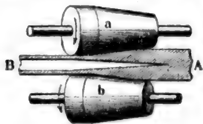
Rohrwalzen.
