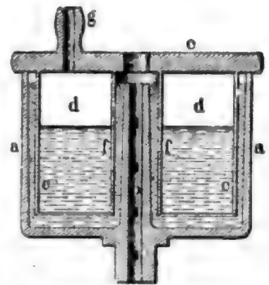
Hambruchs Schmiergefäß.
