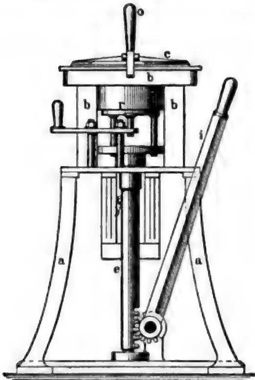
Fig. 3. Neue Teigteilmaschine von Brünig. Vorderansicht.
