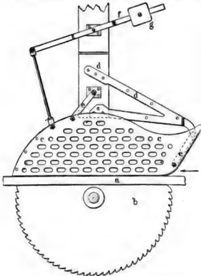
Fig. 1. Schutzvorrichtung an Kreissägen.
