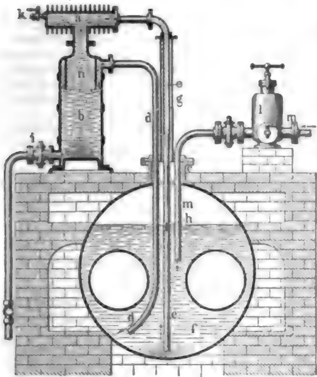
Kesselreinigungsapparat von Derbaug.
