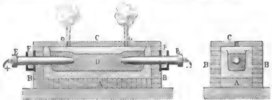
Fig. 2. Längsschnitt. Fig. 3. Querschnitt. Cowles' Apparat zur Darstellung von Aluminium.
