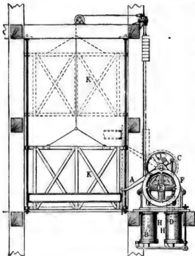
Fig. 4. Selbstthätiger Schachtverschluß von Schüller.
