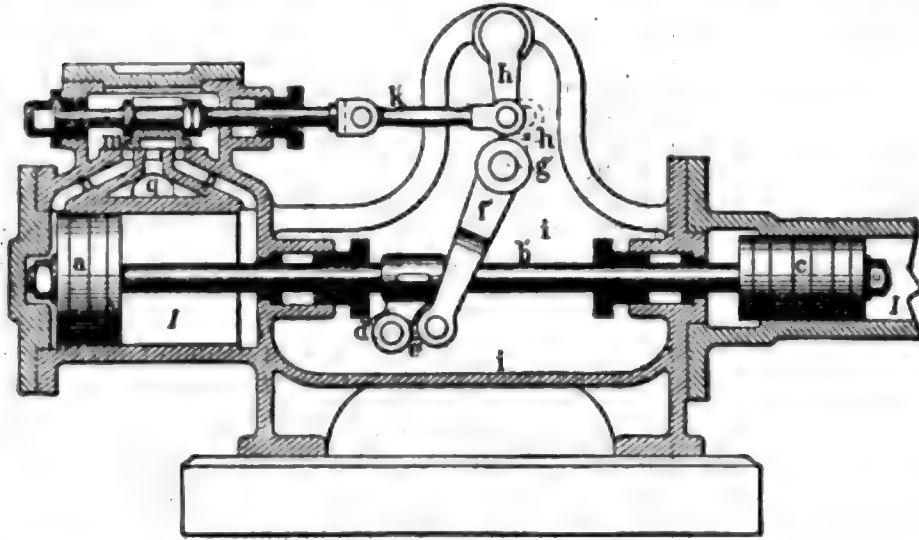
Fig. 1. Längsschnitt. Fig. 1 und 2. Duplex-Pumpe nach Worthingtons System.
