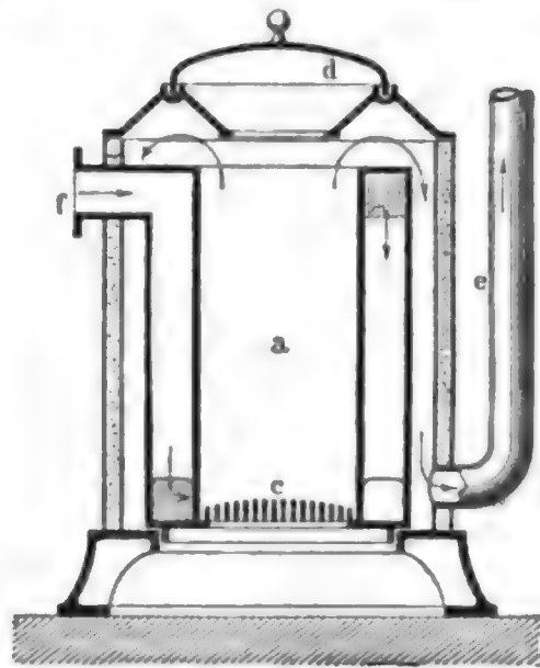
Fig. 1. Vertikalschnitt.
