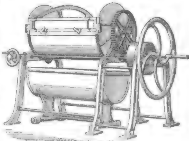
Fig. 1. Knetmaschine von Brüning.
