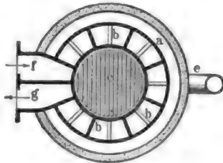
Fig. 2. Horizontalschnitt.
