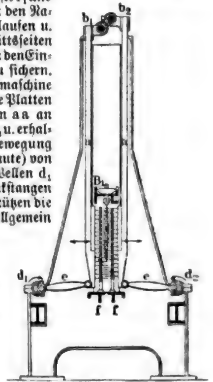
Fig. 2. Stechmaschine.
