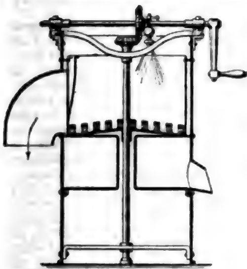
Fig. 1. Durchschnitt. Parff's Kartoffelschälmaschine.
