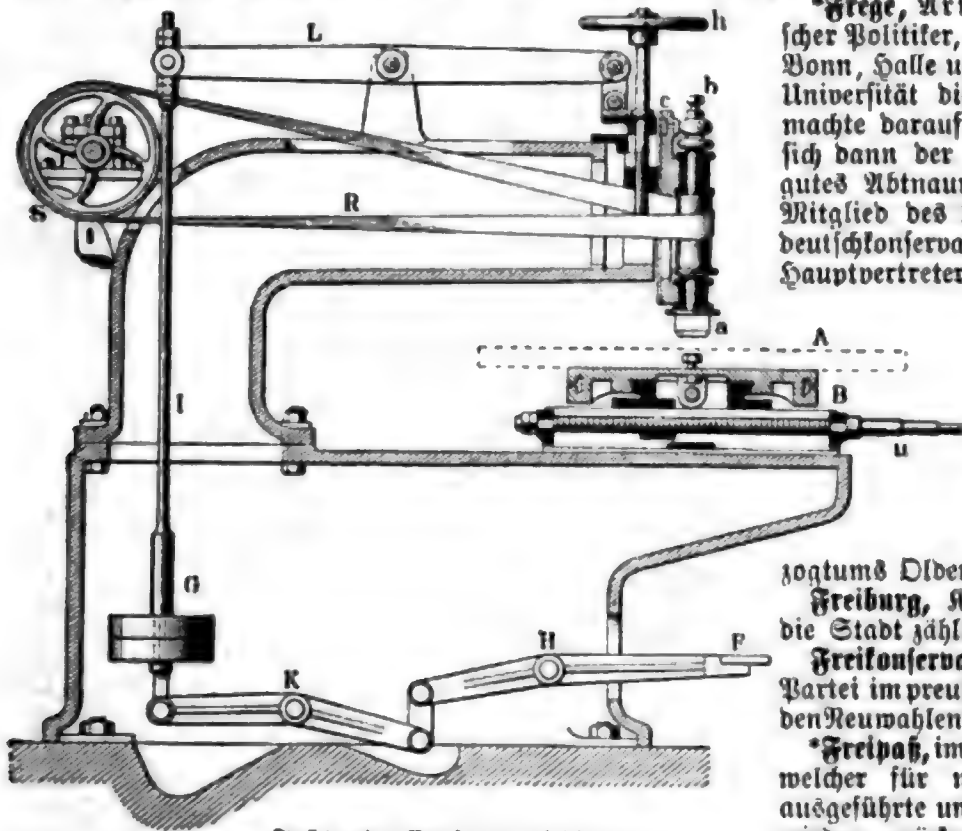
Fräs- oder Versenkmaschine.
