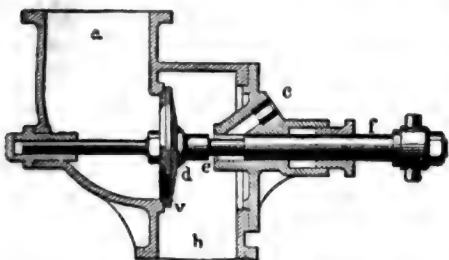
Anfahrvorrichtung von Vorries .
