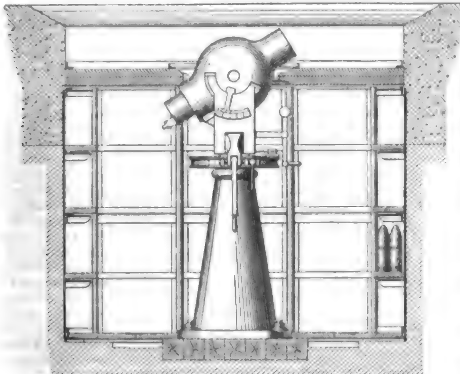
Fig. 2. Panzerstand für 21 cm Mörser.
