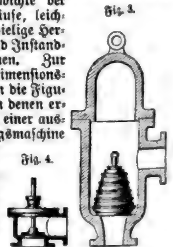
Fig. 3. Selbstthätiges Ventil. Fig. 4. Niedere Ventil. Abmessungen für gleiche Leistung.
