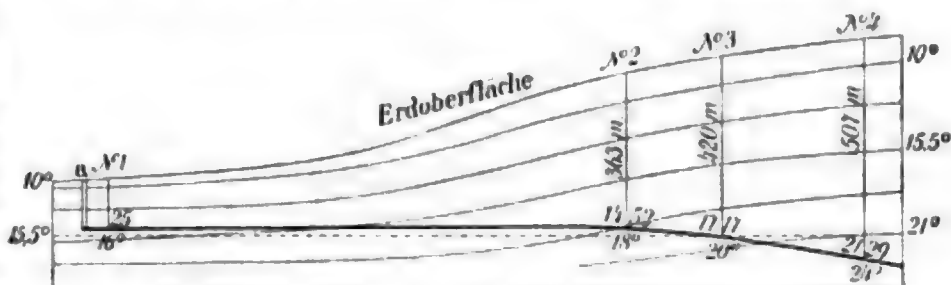
Fig. 1. Verlauf der Isothermen.
