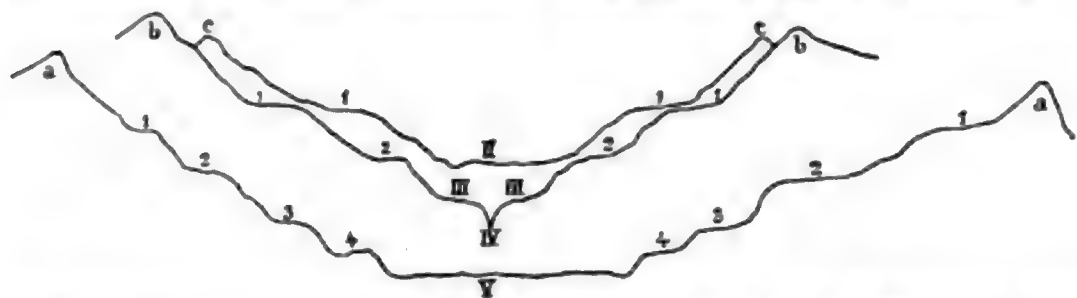
Fig. 3. Querprofil: des Neuzthals nach Heim. a nahe bei Klidorf, b nahe Göschenen, c im Urserenthal. (Die römischen Zahlen bedeuten Thalfufen und die arabischen die ihnen entsprechenden Terrassen.)
