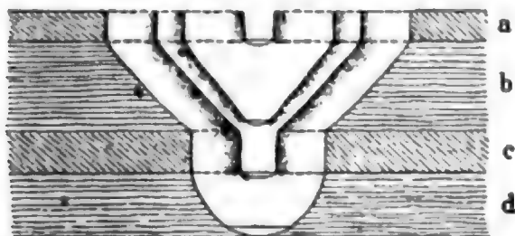
Fig. 2. Querschnitt einer Erosionsrinne.
