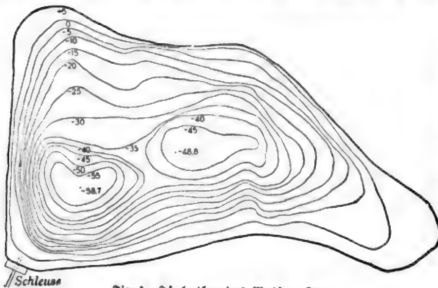
Fig. 1. Isobathen des Weißen Sees.
