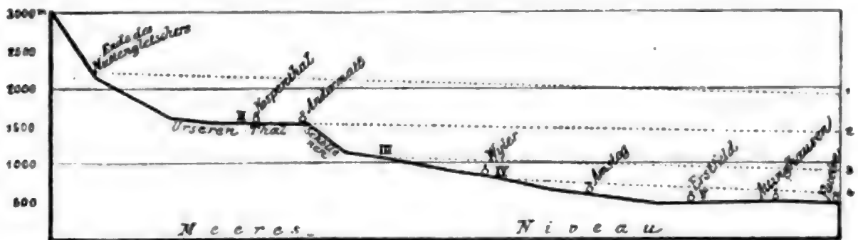
Fig. 2. Längendurchschnitt durch das Neuzthal. Höhenmaßstab fünfmal größer als der Längenmaßstab.
