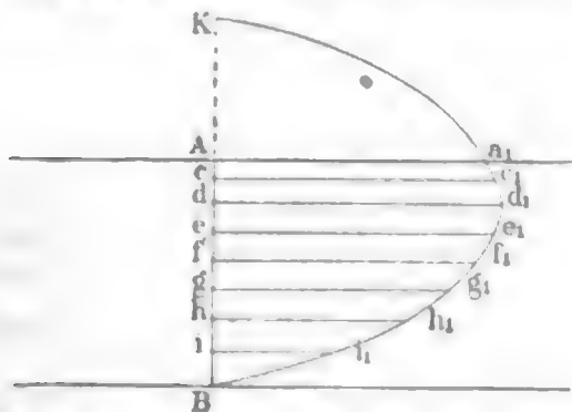
Fig. 2 Geschwindigkeit der einzelnen Stromschichten.
