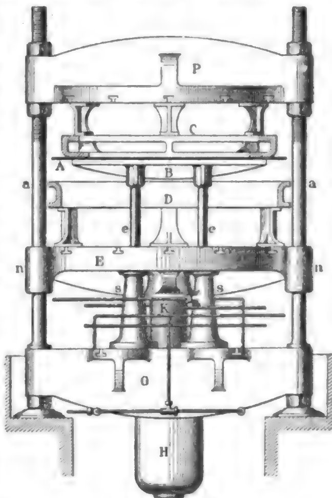
Bördelpresse.
