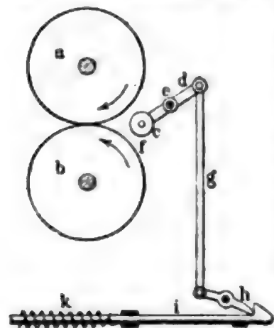
Eisdrähtige Ausrückung der Kalanders.
