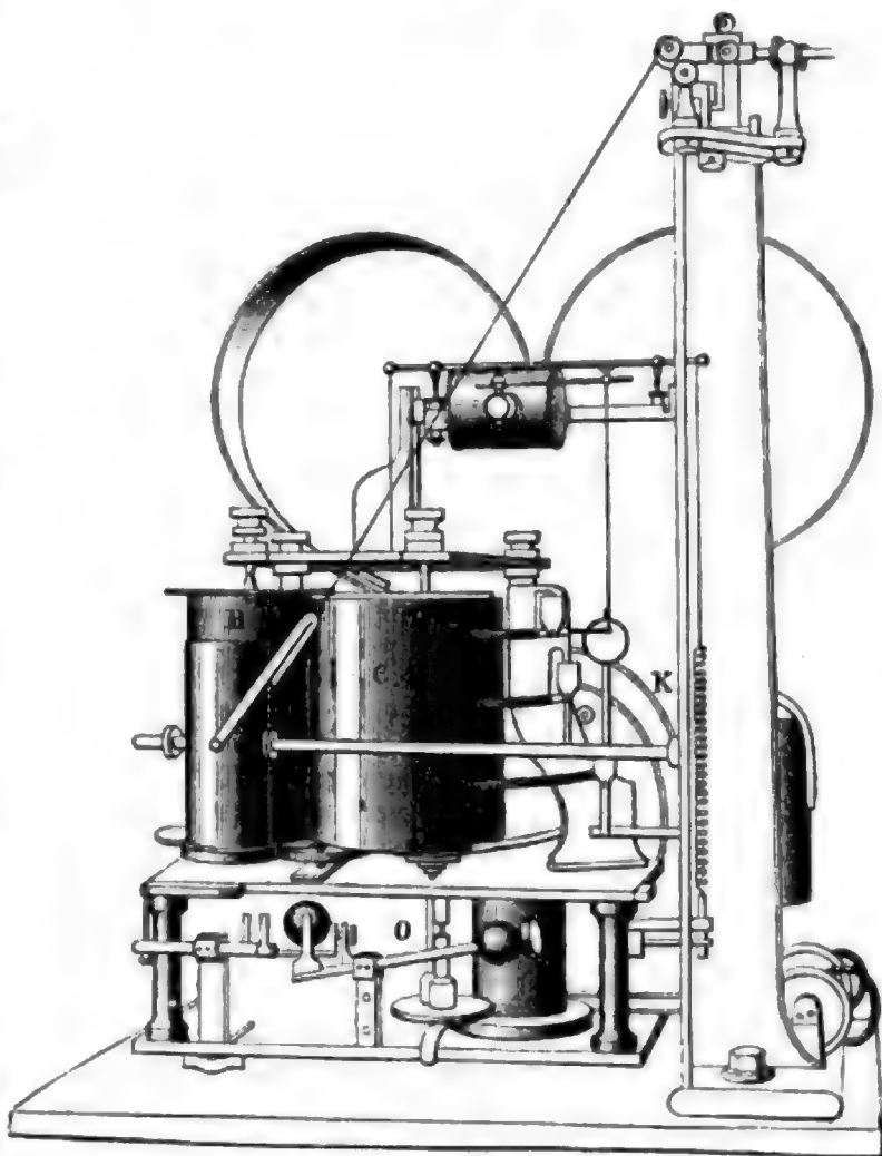
Seismograph von Gray und Milne.
