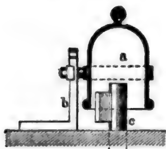
Fig. 4. Schutzglocke an Fräsemaschinen.
