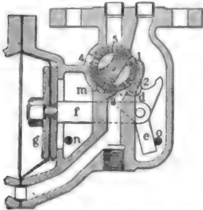
Fig. 3. Funktionsventil der Carpen-terischen Schnellbremse
