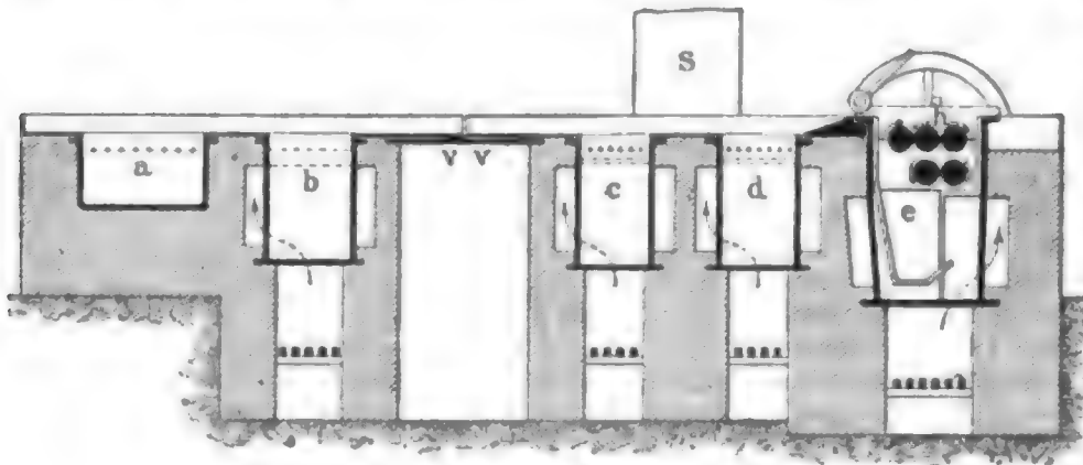
Fig. 2. Längsschnitt.
