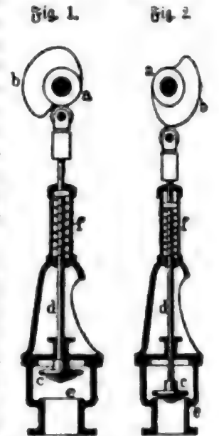
Fig. 1 u. 2 Niedere Ventil mit Zwangschluß
