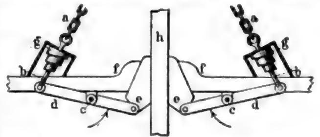
Fig. 1. Keilfangvorrichtung von Libotte.
