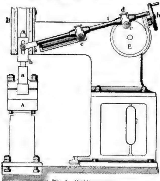
Fig. 1. Lufthammer.
