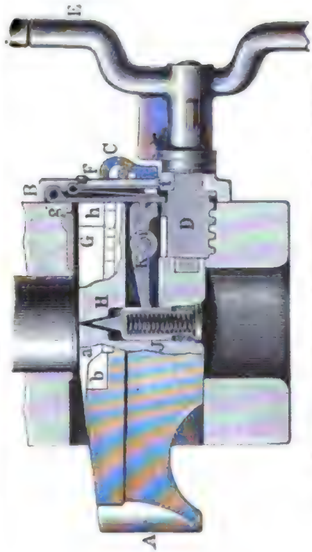
Fig. 3. Krupp'scher Horizontalkeilverschluss für Schnellfeuerkanonen, in der Mitte wagerecht durchgeschnitten.
