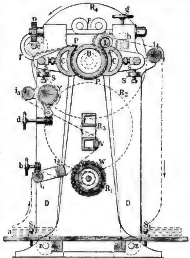
Muldenkalander.
