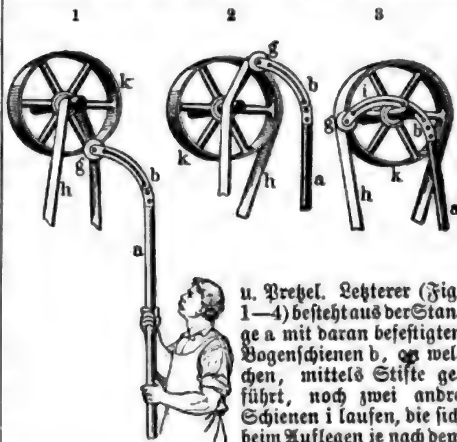
Fig. 1—3. Drehels Riemenaufleger.
