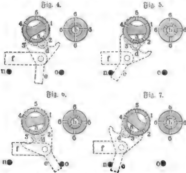
Fig. 4-7. Verschiedene Stellungen des Funktionsventils.
