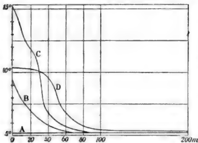
Fig. 2. Kurven der Temperaturveränderungen.
