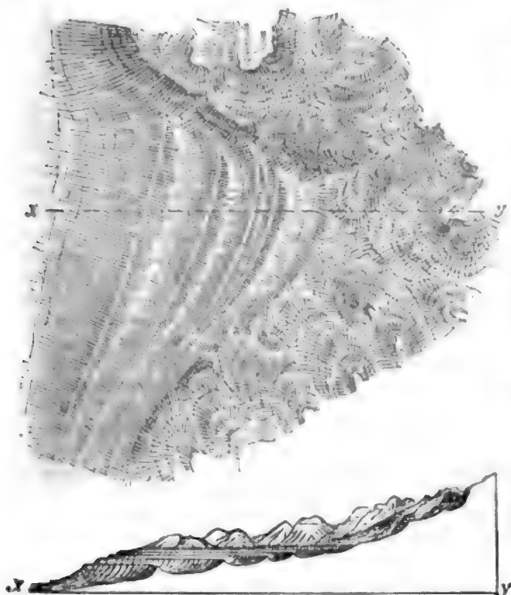
Fig. 3a. Querschnitt. Fig. 3 und 3a. Barrenbildung.
