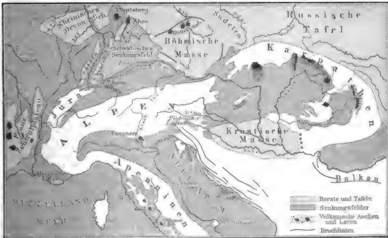
Fig. 3. Der Hauptstamm der Alpen (nach G. Suez).
