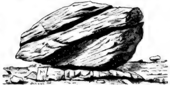
Fig. 1. Erratischer Block aus Silurschiefer (2m × 3,5m) bei Clapham in Northshire.
