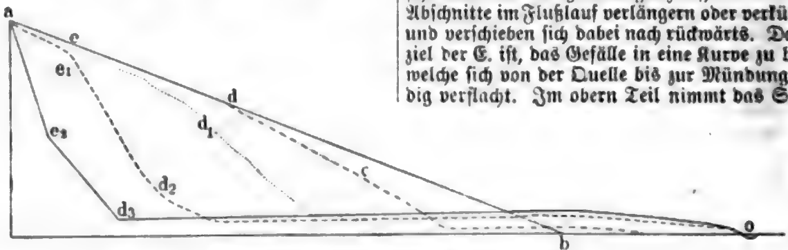
Fig. 1. Bängenprofil einer Erosionsrinne.
