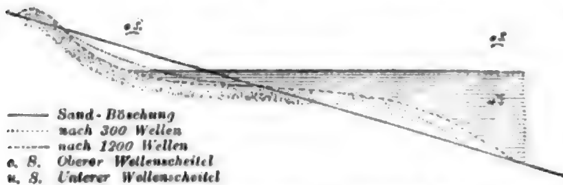
Fig. 1. Strandbildung bei weichem Gestein.
