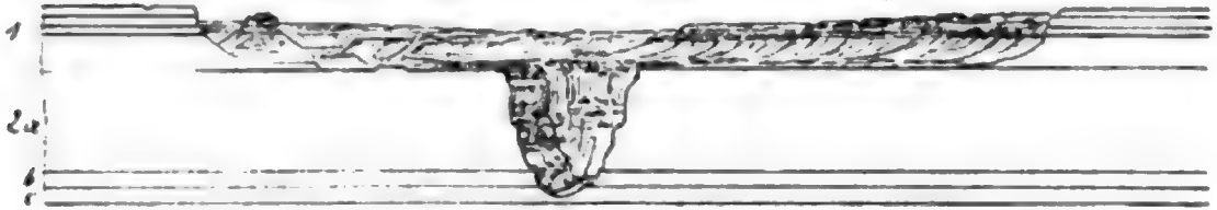
Fig. 1. Querprofil durch den Cañon des Colorado.
