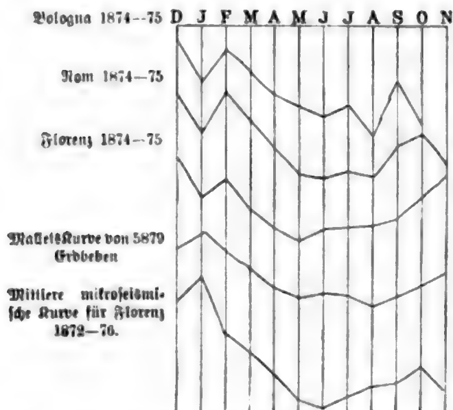
Fig. 4. Monatskurven der mikroseismischen Störungen.
