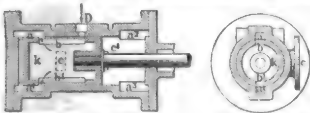
Fig. 1. Längsschnitt. Fig. 2. Querschnitt. Fig. 1 u. 2 Gräbner-Maschine.
