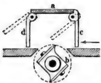
Fig. 5. Schutzvorrichtung an Hobelmaschinen.
