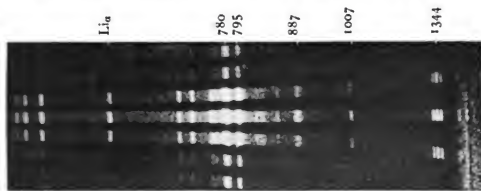
Fig. 6. Gekreuzte Spektren.
