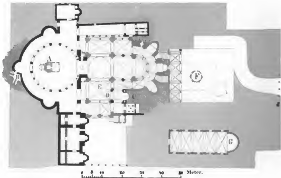
Grundriß der Kirche des heiligen Grabes.
