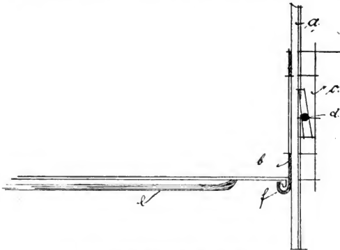
Fig. 3. Vorderansicht des Schildes mit Boden.
