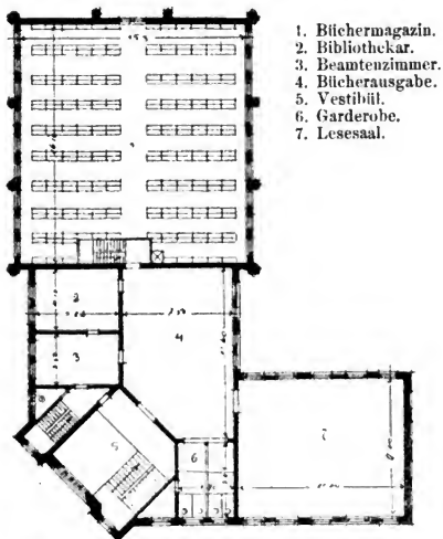
Stadtbibliothek Danzig. Grundriß II: Obergeschoss. Maßstab 1 : 400 = 2 1/2 mm : 1 m.
