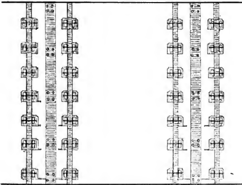
Danziger Büchergestell Steeg. Fig. 5. Seitenansicht eines Binderfeldes.
