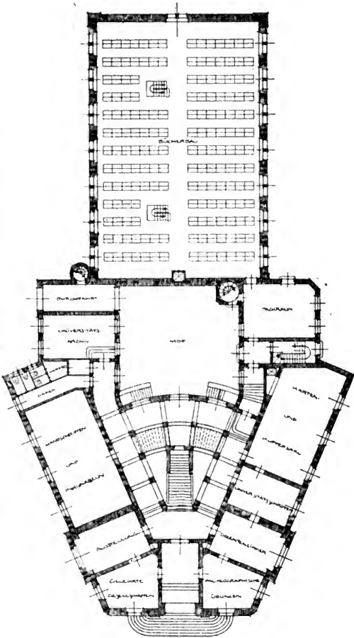
Universitätsbibliothek Gießen. Erdgeschoss. Maßstab 1 : 400 = 2½ mm : 1 m.
