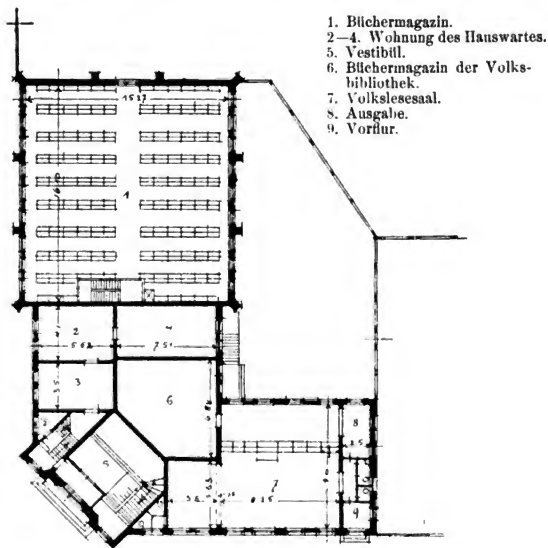
Stadtbibliothek Danzig. Grundriß I: Erdgeschoss.
