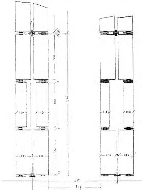
Danziger Büchergestell Steeg. Fig. 4. Grundriß eines Binderfeldes.
