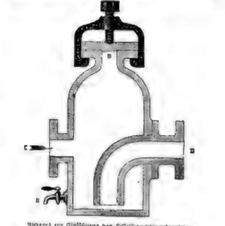
Apparat zur Einführung von Rostlötlösungen.
