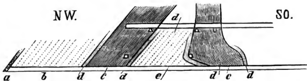
Profil eines Sattels der Braunkohlengrube „Präsident“.
