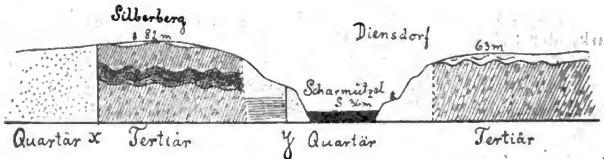
Schematisches Profil durch den Scharmützel-See bei Fürstenwalde.
