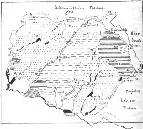
Geognostische Skizze des Barnim-Plateaus.
