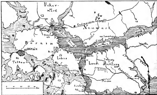
Die Nachbarschaft des Oderbruch-Grabens.
