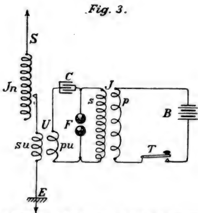
B Batterie; C Kondensator; E Erde; F Funkenstrecke; J Induktorium ( p primäre, s sekundäre Spule); J n Regulierbare Selbstinduktionspule; U Transformator oder Uebertrager ( pu primäre, su sekundäre Spule); T Taste.
