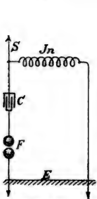
C Kondensator; F Funkenstrecke; J_n Selbstinduktionsspule S Senderdraht.
