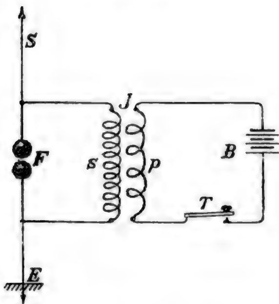
B Batterie; E Erde; F Funkenſtrecke; J Induktorium ( p primäre, s ſekundäre Spule); S Senderdraht; T Taſte.
