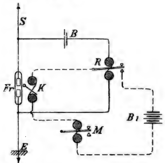
B u. B1 Batterien; E Erde; Fr Fritter; K Klopfer zum Entſritzen; M Morſeſchreiber; R Relais; S Empfängerdraht.
