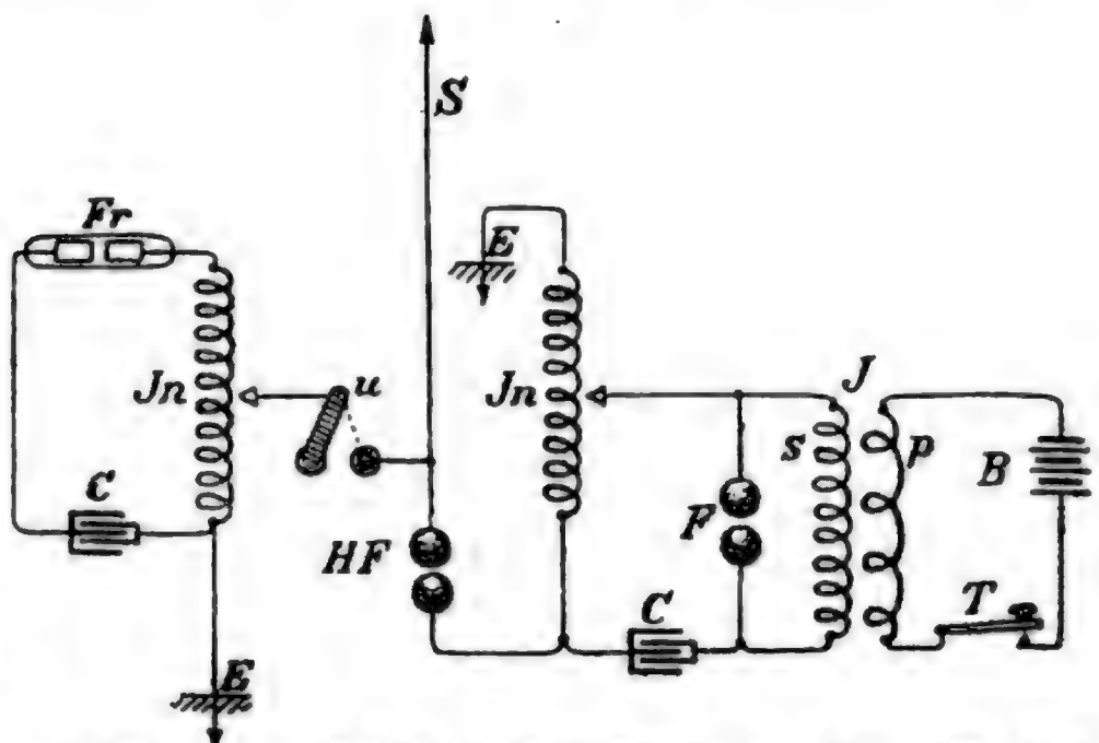
C Kondensator; E Erde; F Funkenstrecke; Fr Fritter; HF Hilfsfunkenstrecke; J_n Regulierbare Selbstinduktionsspule; S Sender- bzw. Empfängerdraht; u Umschalter.
