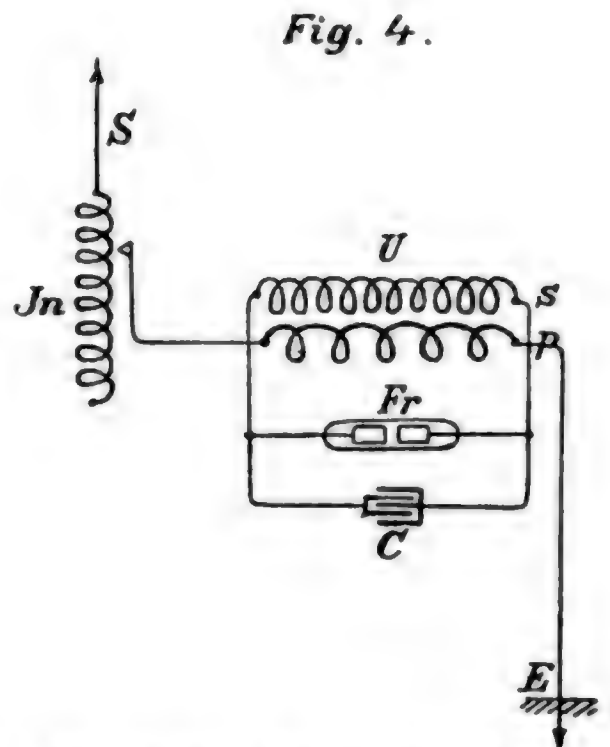
C Regulierbarer Kondensator; E Erde; Fr Fritter; J n Regulierbare Selbstinduktionspule; U Uebertrager ( p primäre, s sekundäre Spule).
