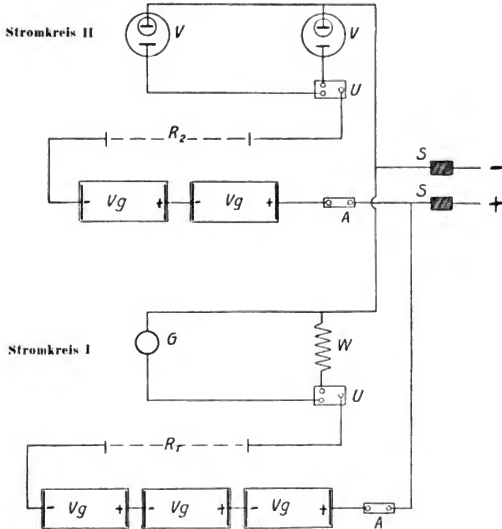
Schaltungsskizze.
