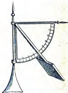
Windmesser von Hoop.
