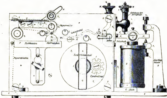
Morseapparat. Aus Hamacher, Telegraphie und Telephonie.
