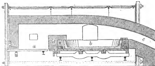
Längsdurchschnitt durch einen Quadelofen. Aus Binz, Kohle und Eisen
