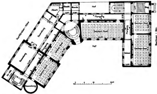
Sowjetgeschloß.
