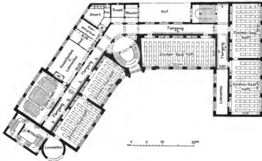
Obergeschoss.
