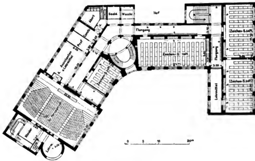
Erdgeschloß.
